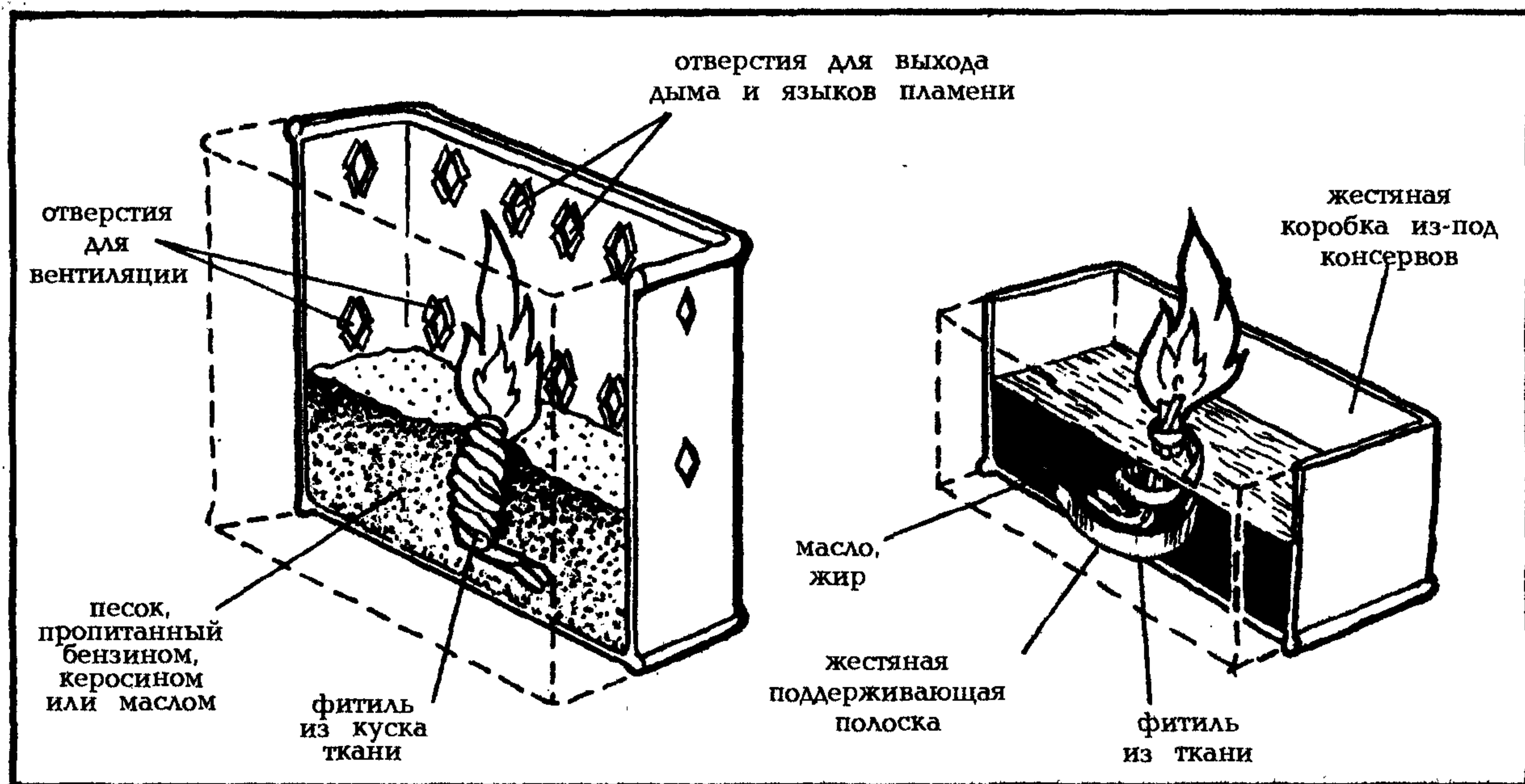
Рис. 74. Печи, изготовленные из металлических емкостей.
