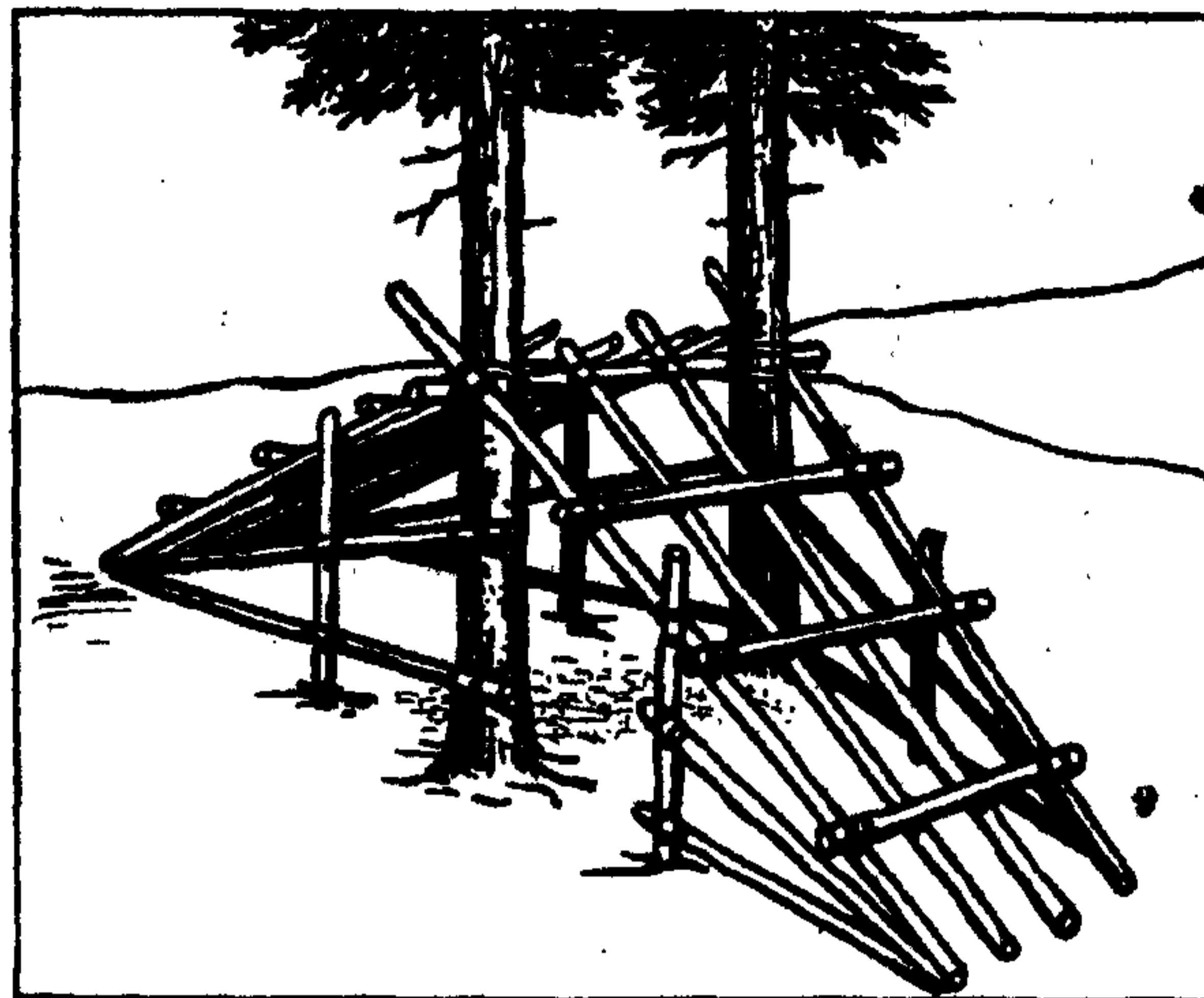
Рис. 44. Навес с двускатной крышей (каркас).
