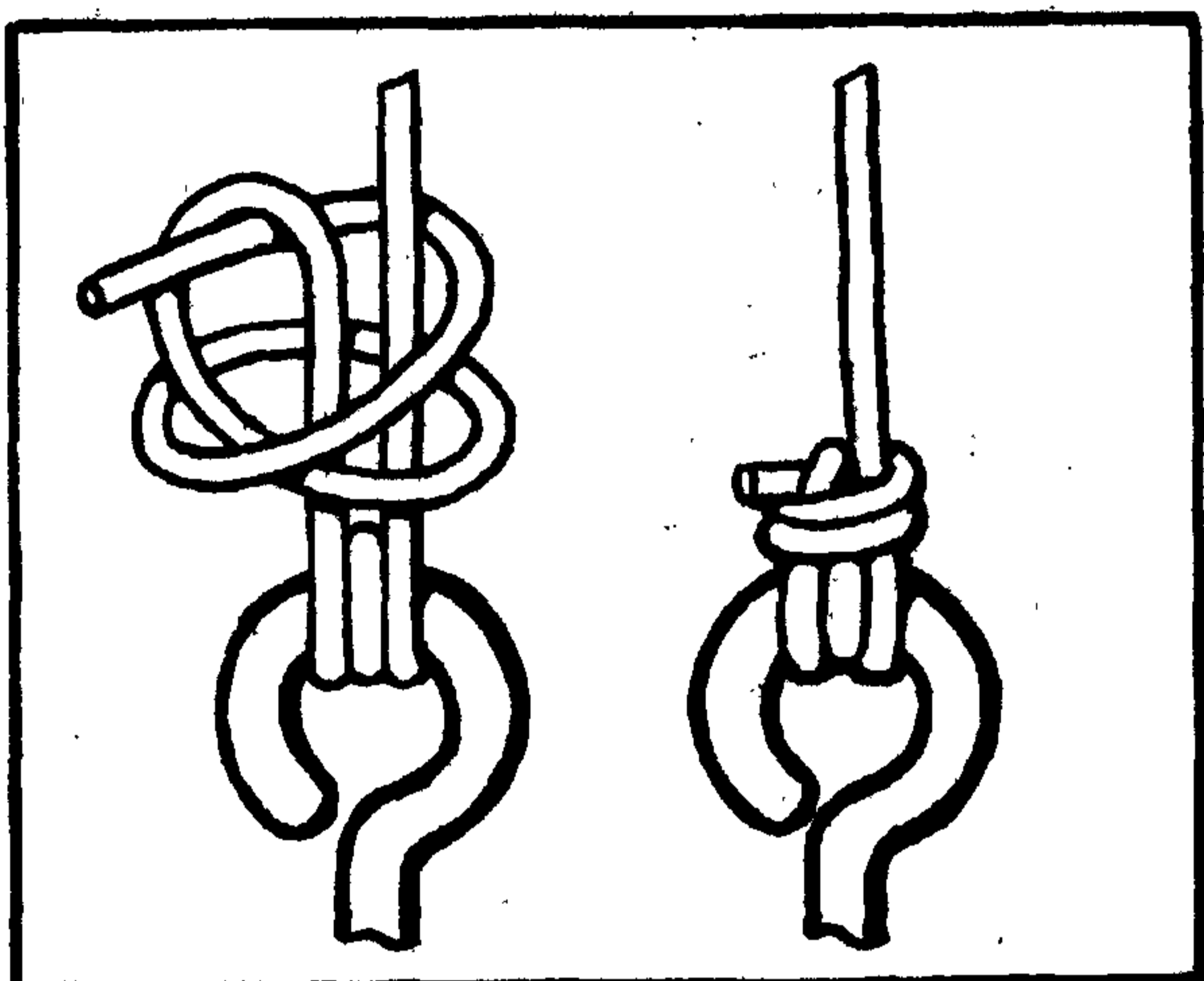
Рис. 113. Узел с обвивом колечка и иетли.
