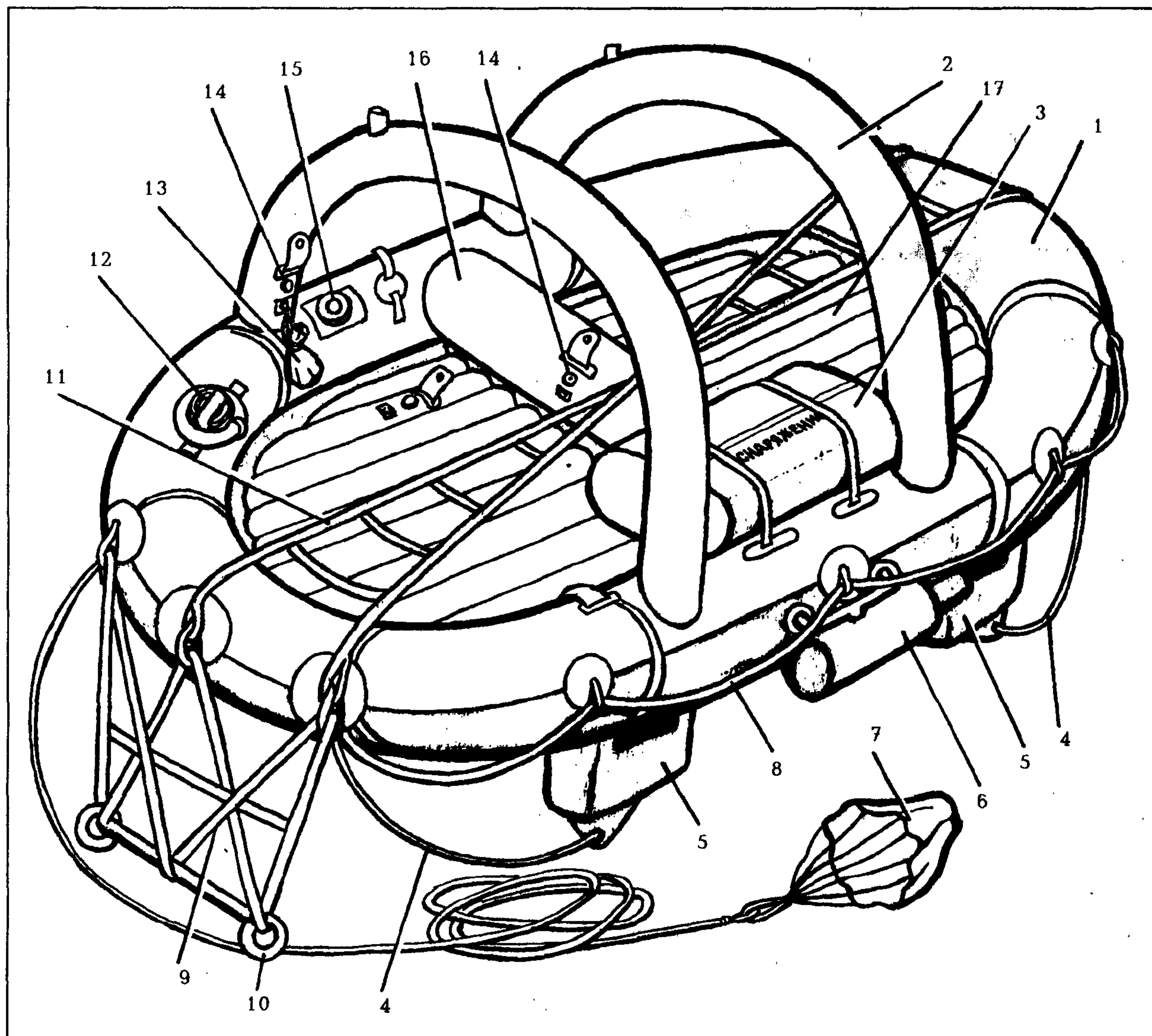
Рис. 282. Устройство плота ПСН-6 (тент условно снят):
