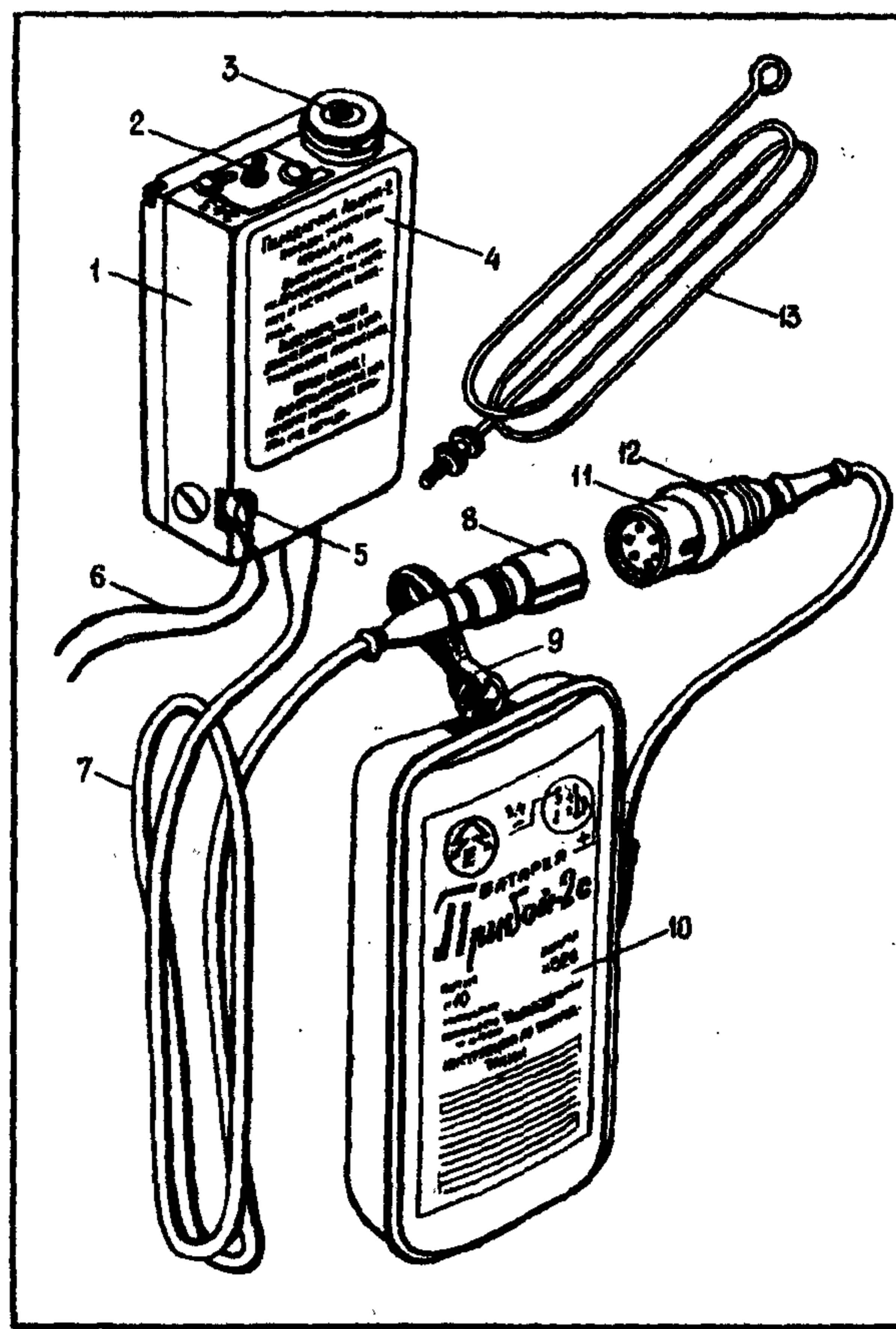
Рис. 265. Автоматический малогабаритный радиомаяк "Авария-2":
