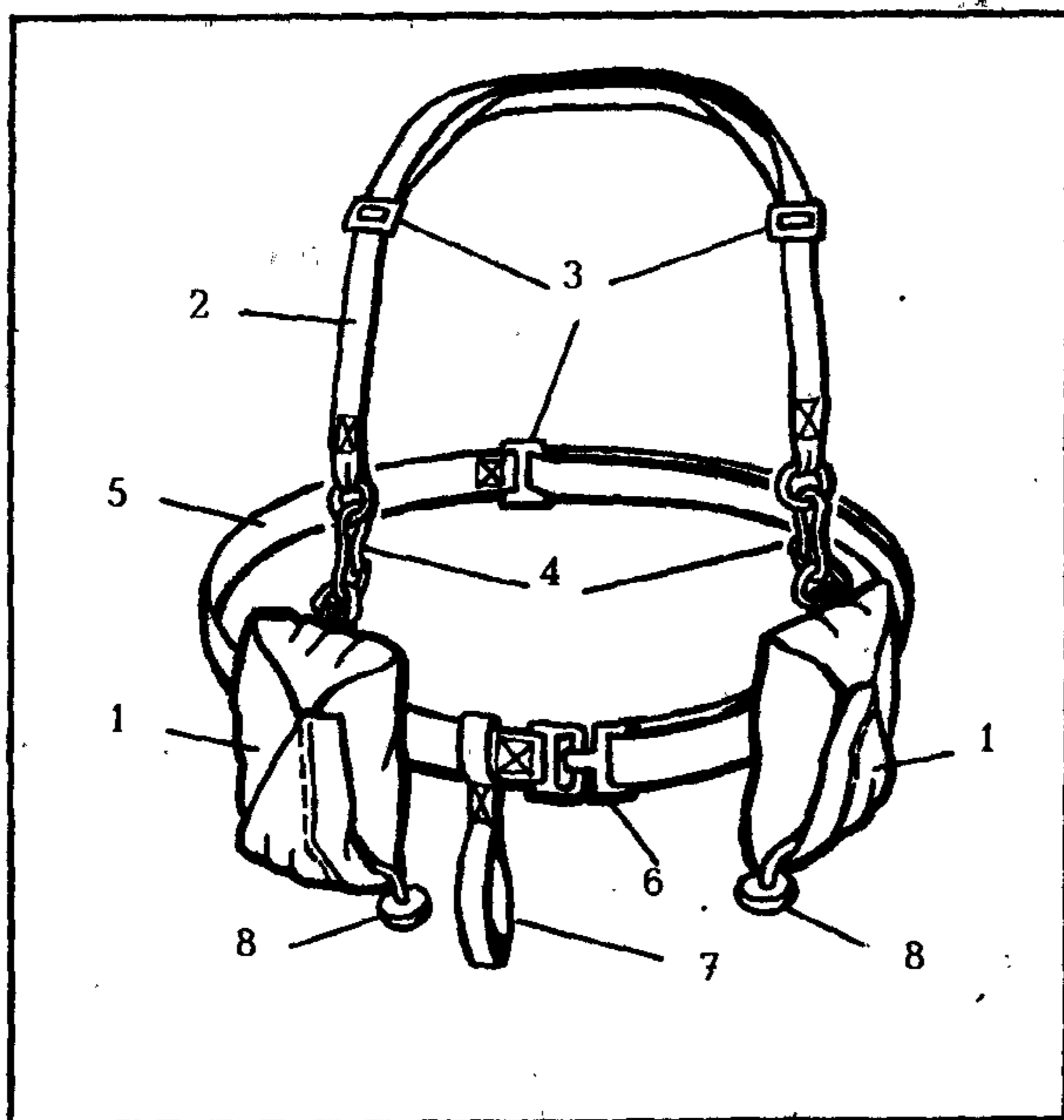
Рис. 276. Спасательный пояс АСП-74:
