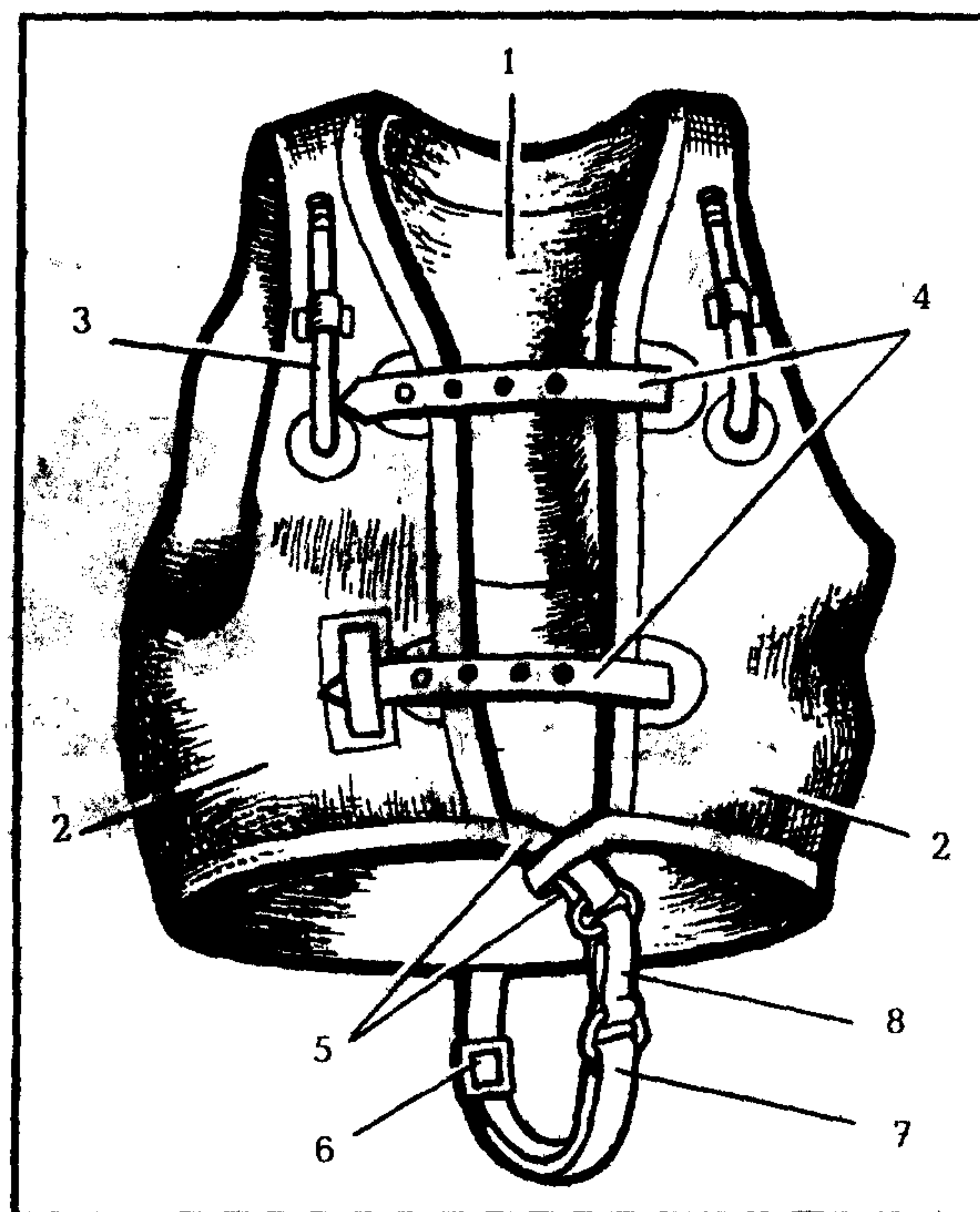
Рис. 272. Спасательный жилет САЖ-43П:
