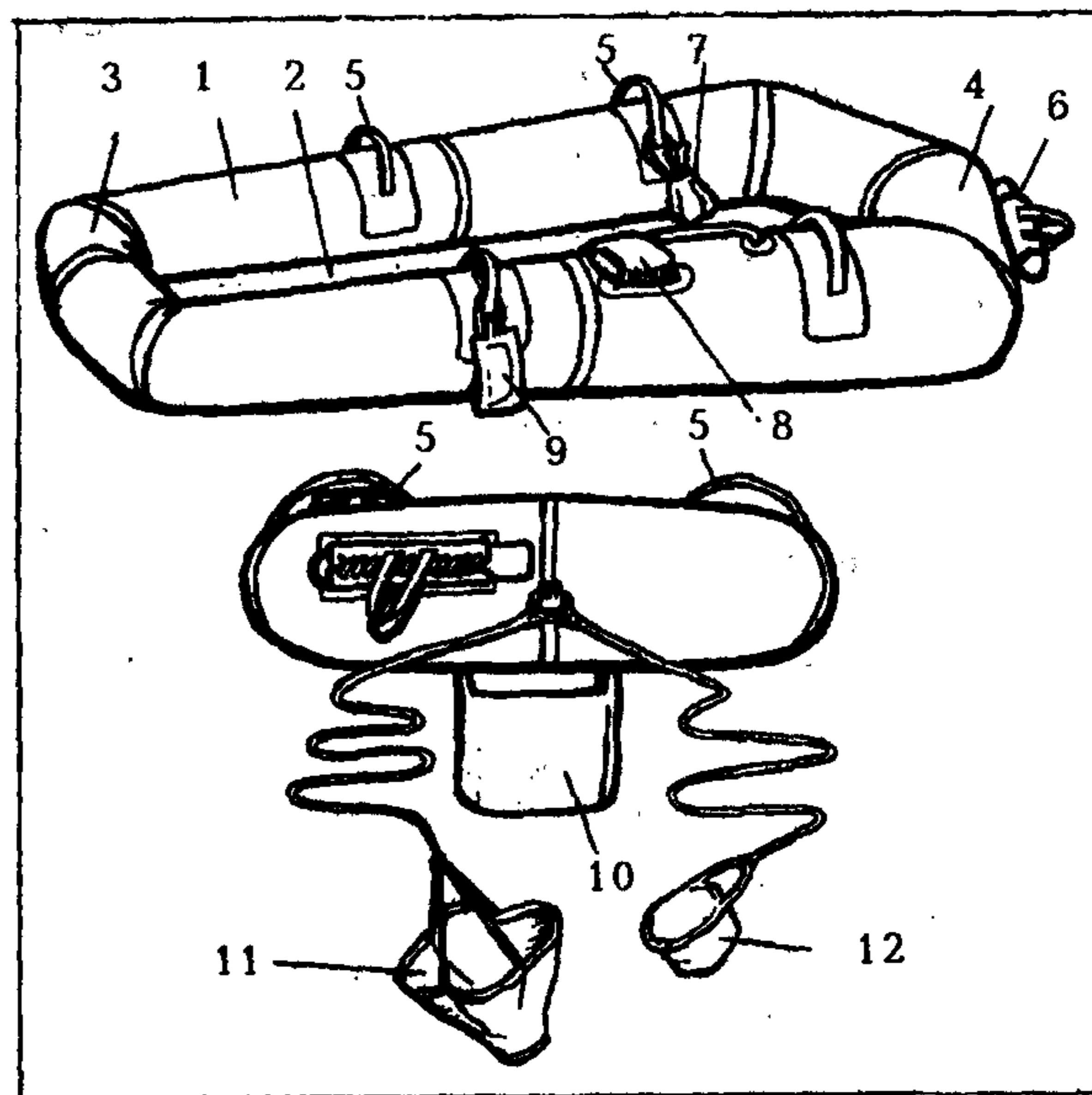
Рис. 277. Спасательная лодка МЛАС-1 "ОБ":
