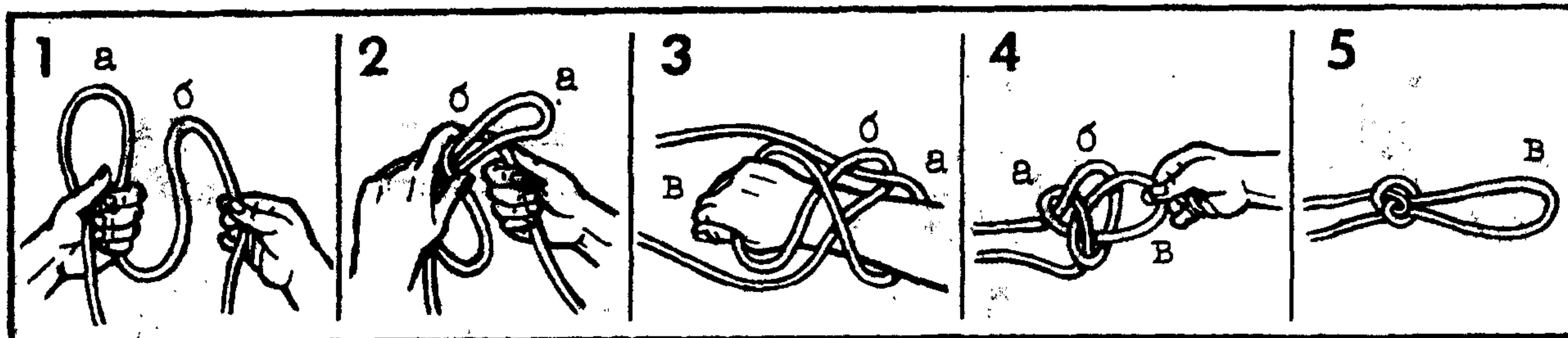
Рис. 213. Такелажный узел.
