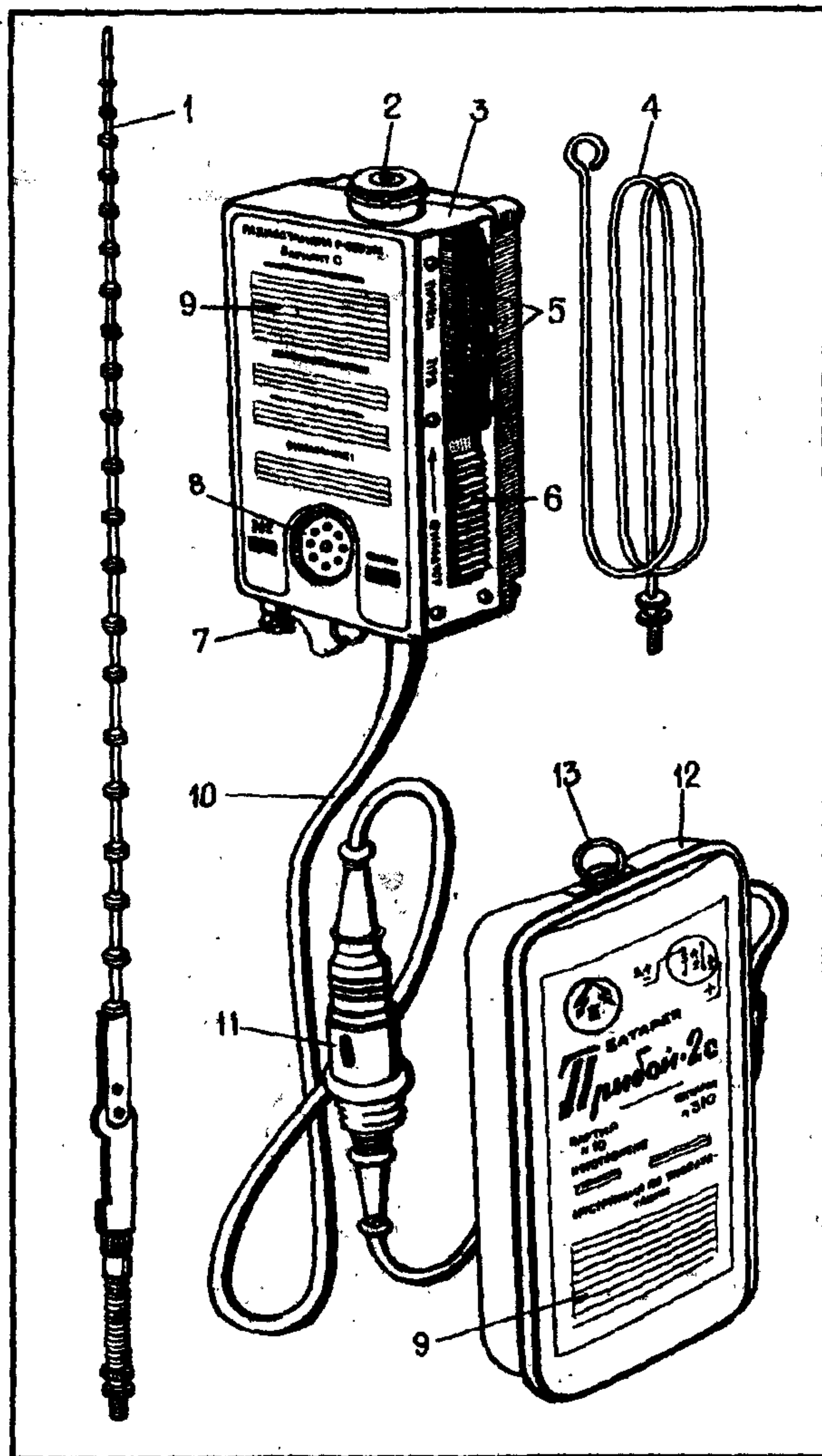
Рис. 261. Радиостанция Р-855УМ:
