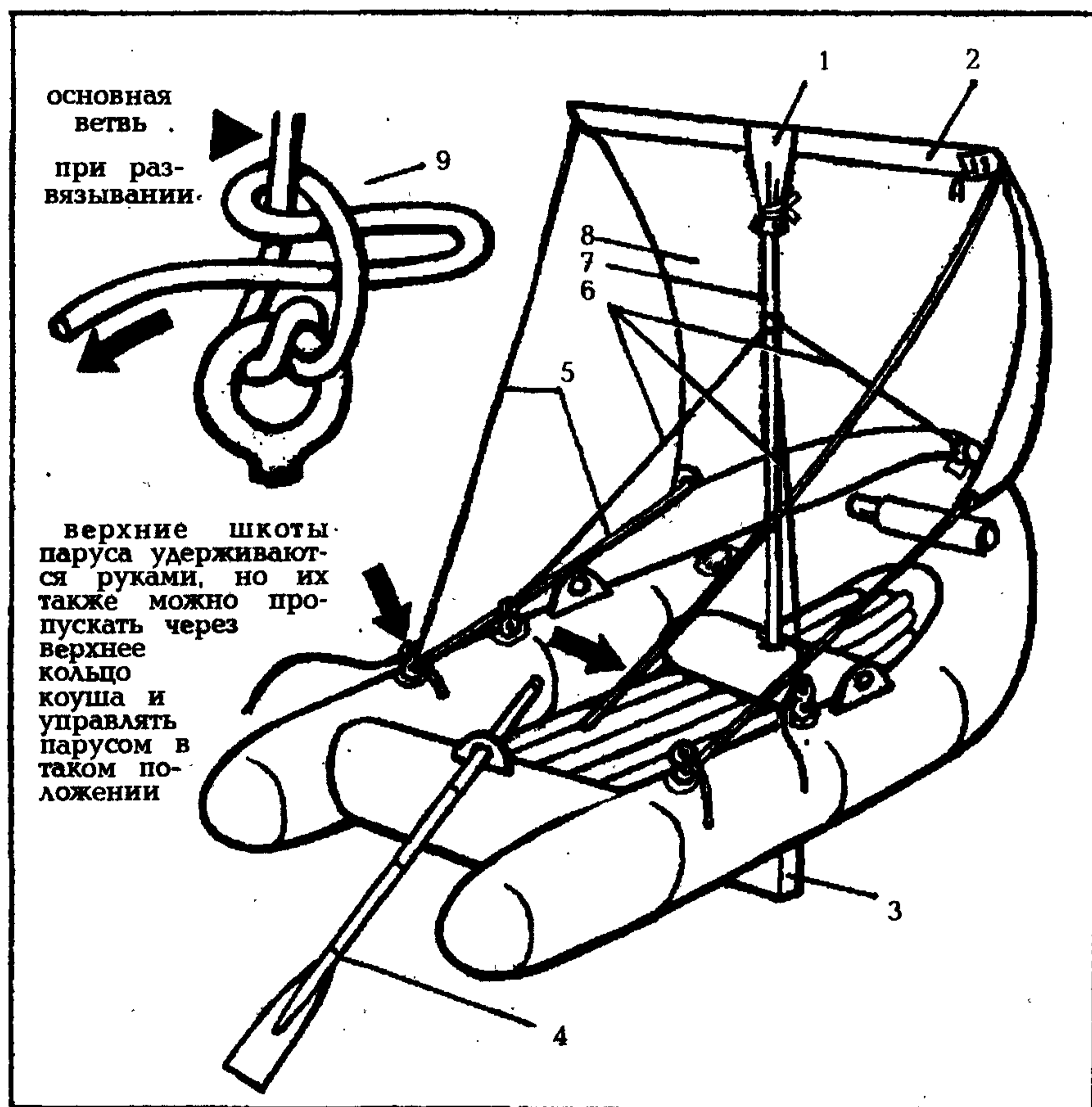
Рис. 280. Лодка ЛАС-5М-3, оборудованная в парусном варианте:
