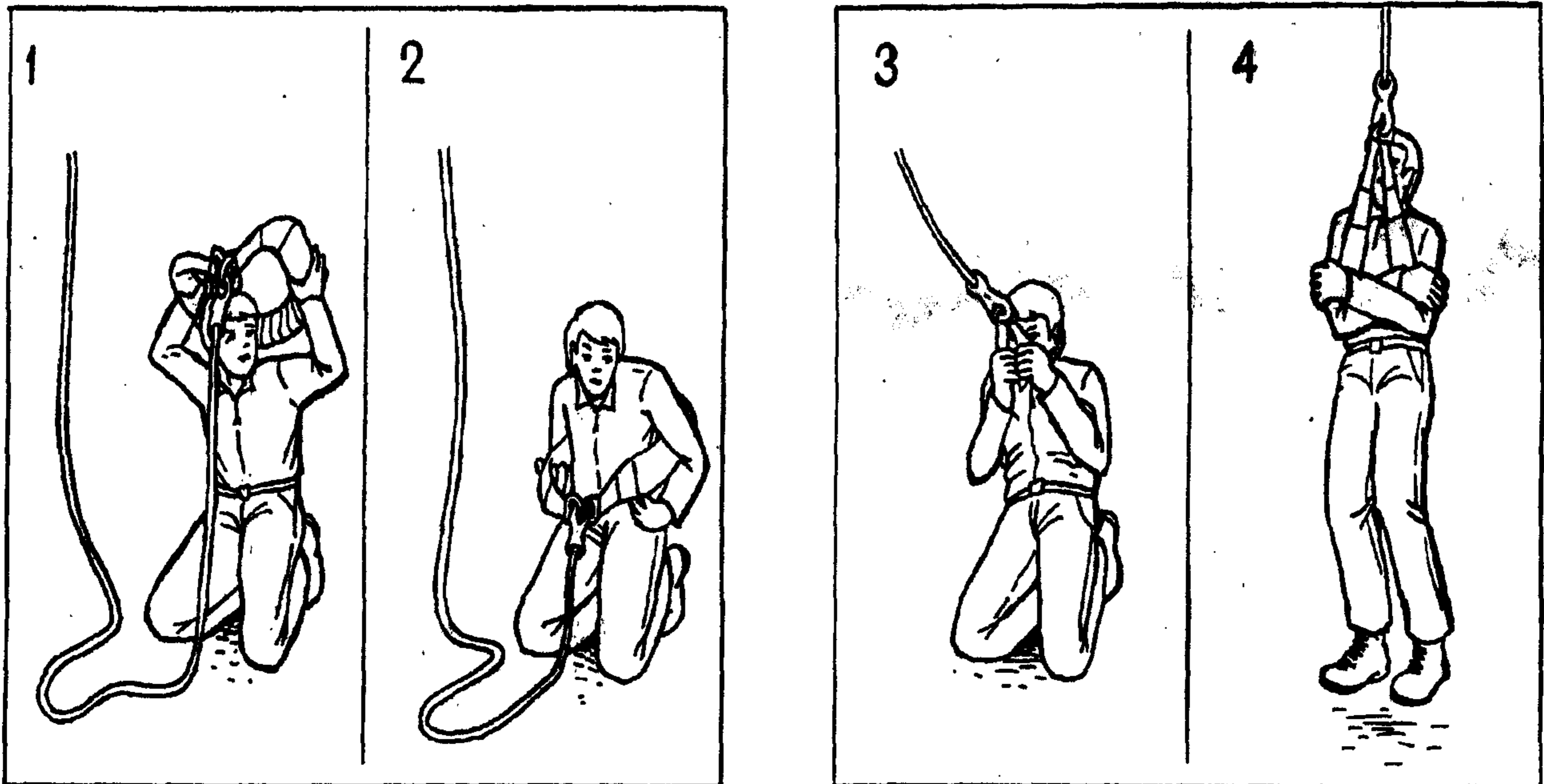
Рис. 303. Подъемный пояс и правила его применения.
