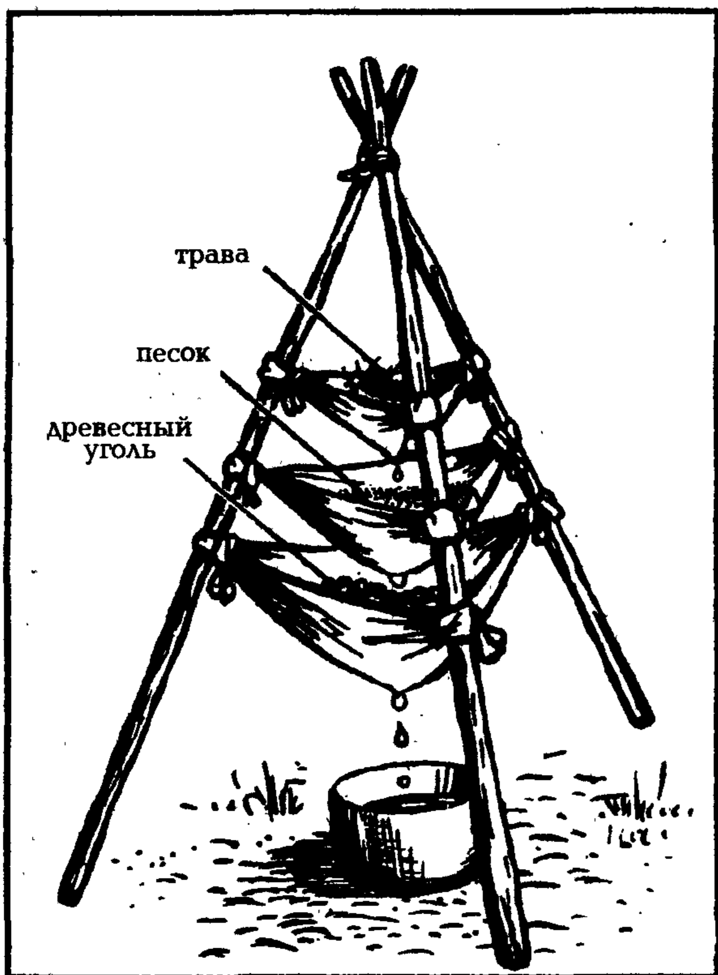
Рис. 86. Фильтрация воды.
