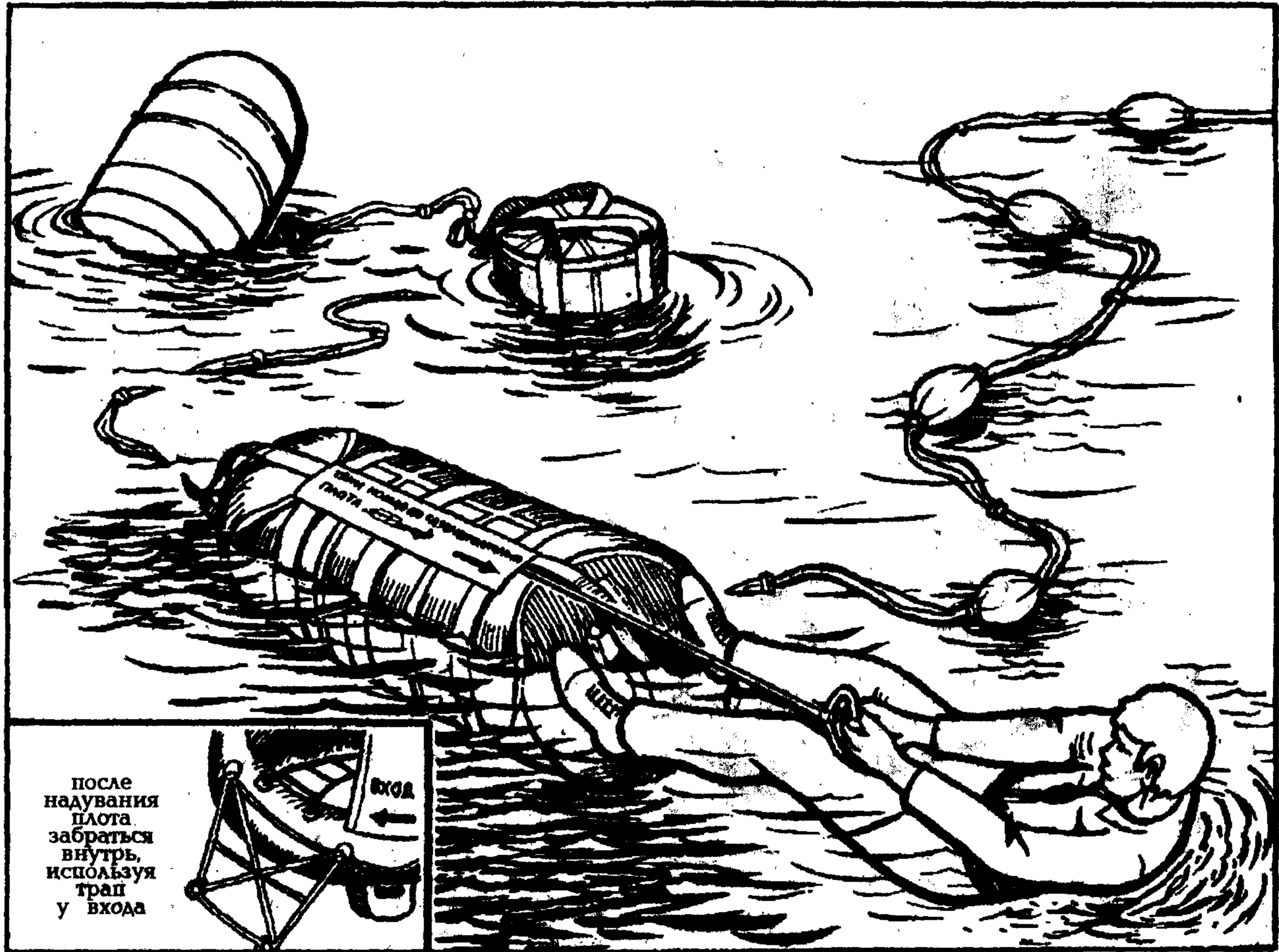
Рис. 260. Включение системы надувания плота и раскрытия упаковки.
