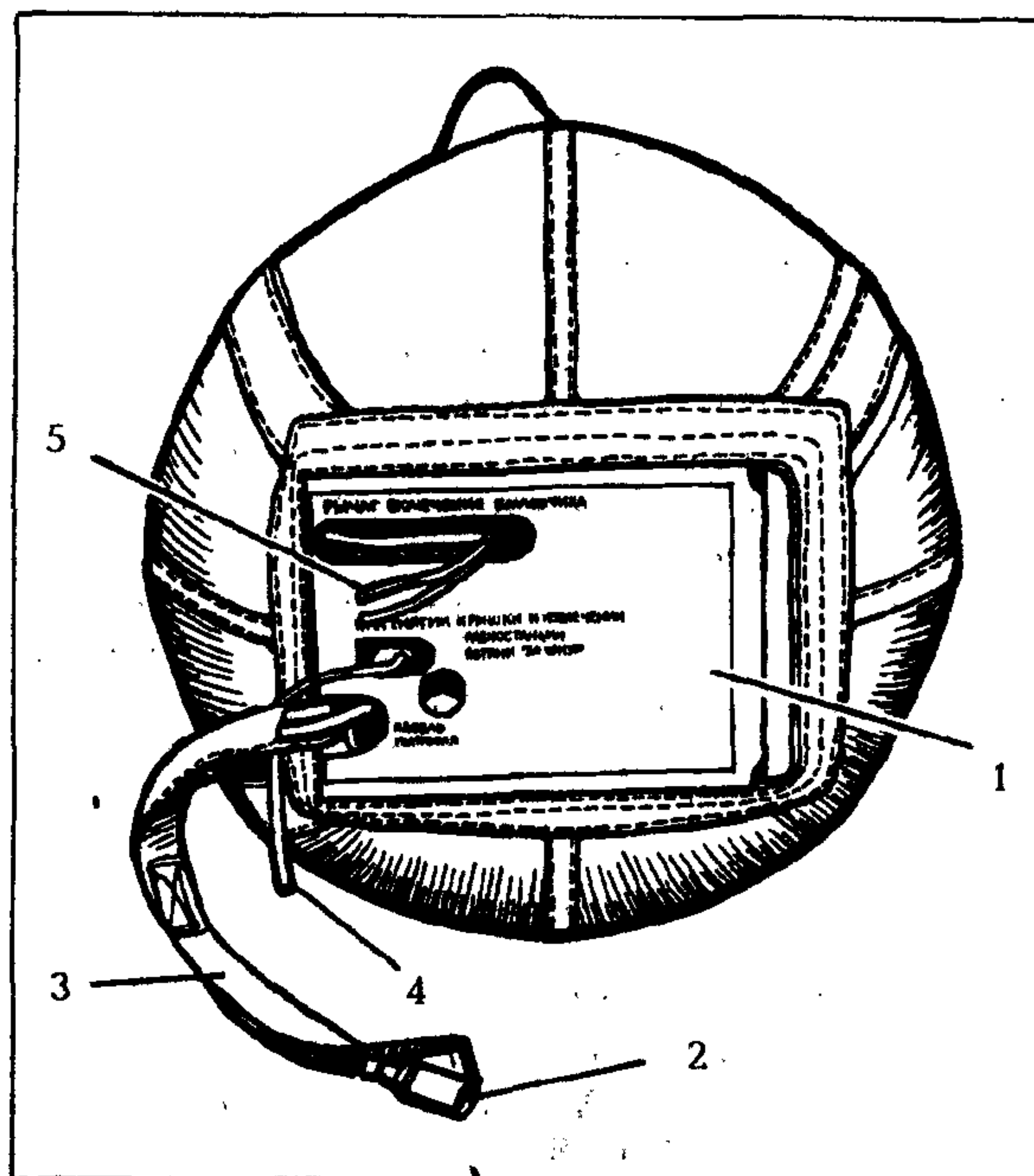
Рис. 263. Вид радиомаяка "Комар-2М" снизу:
