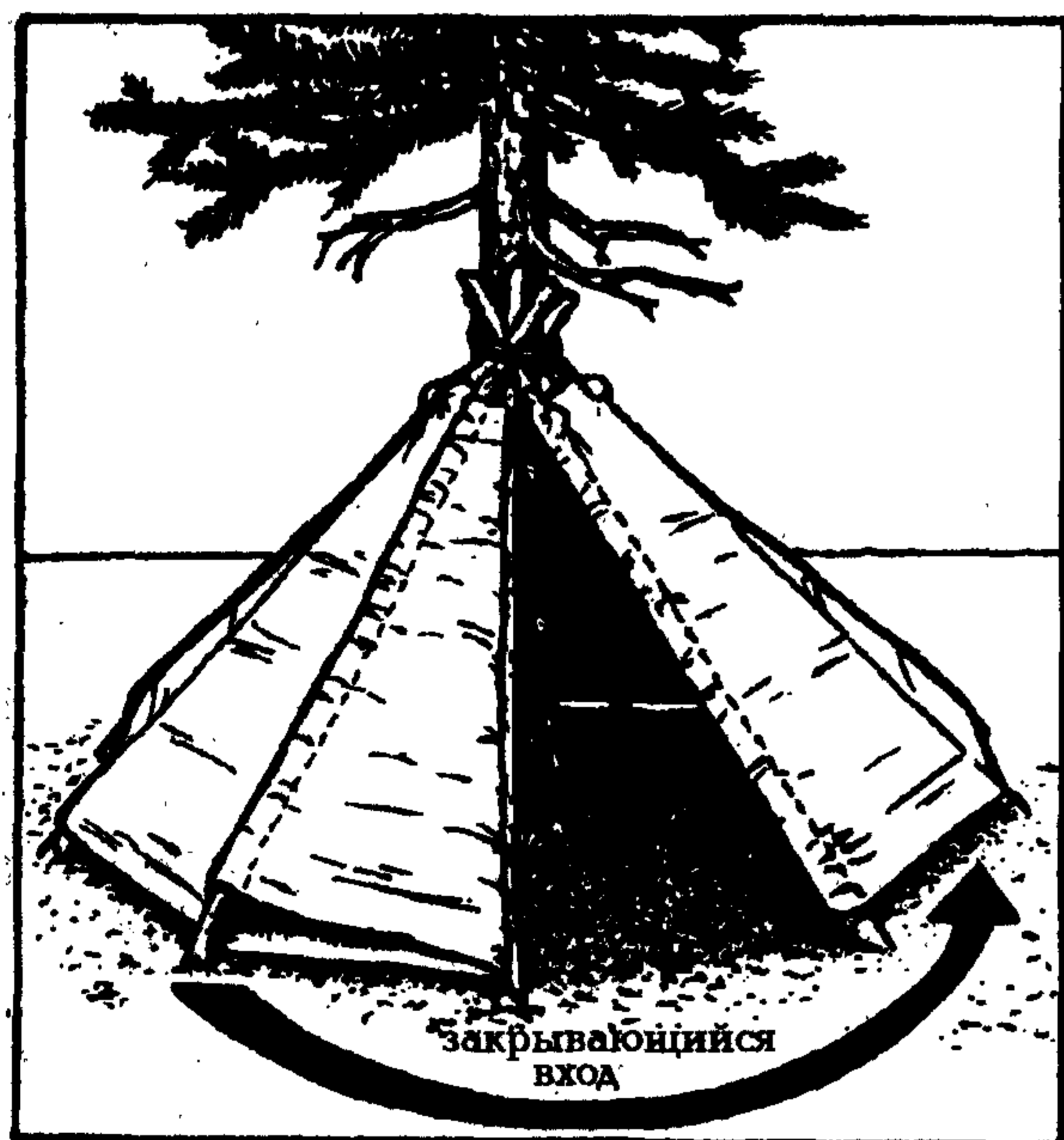
Рис. 39. Круглый шалаш из ткани, построенный вокруг дерева.
