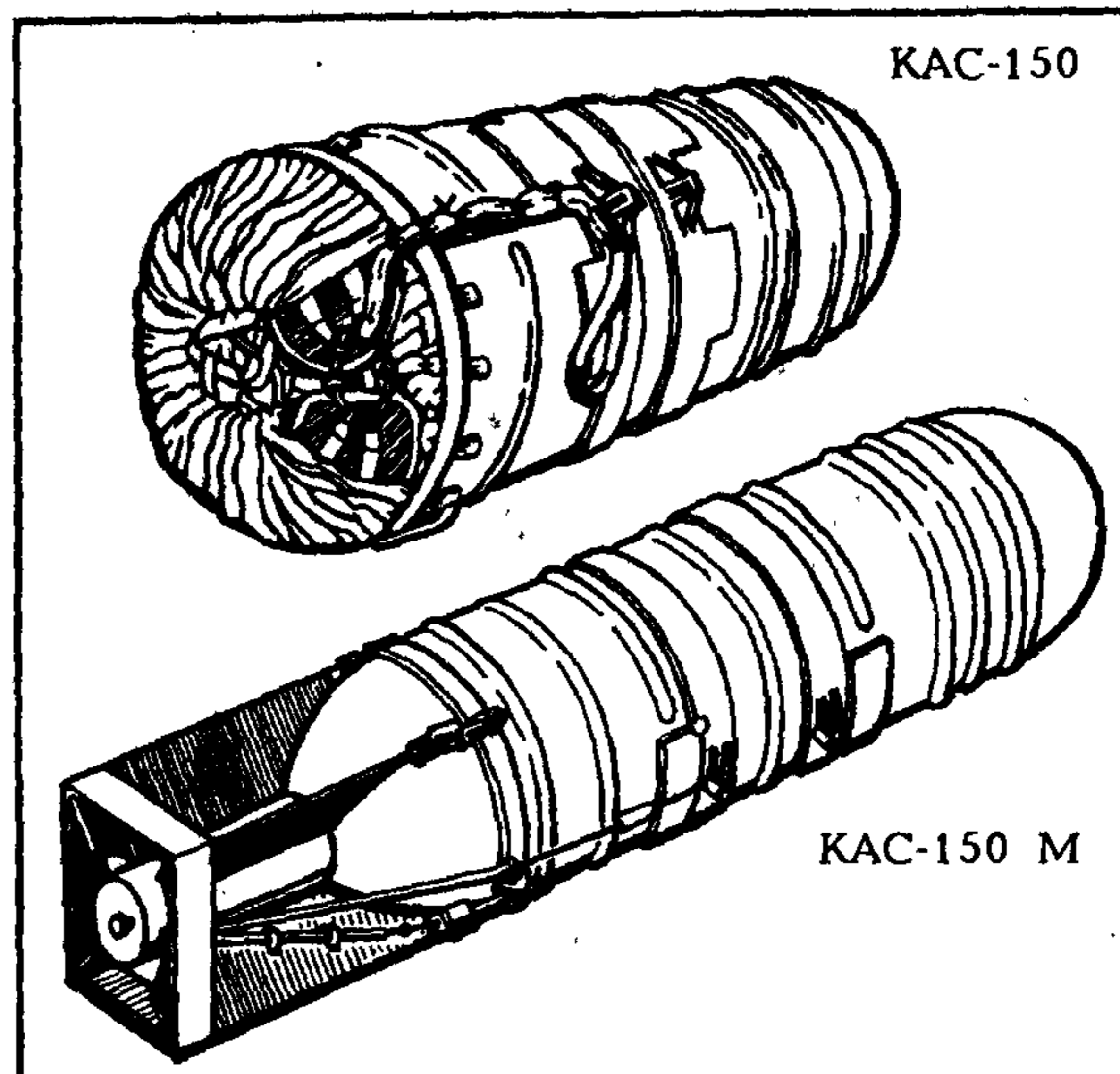
Рис. 257. Общий вид спасательных контейнеров.
