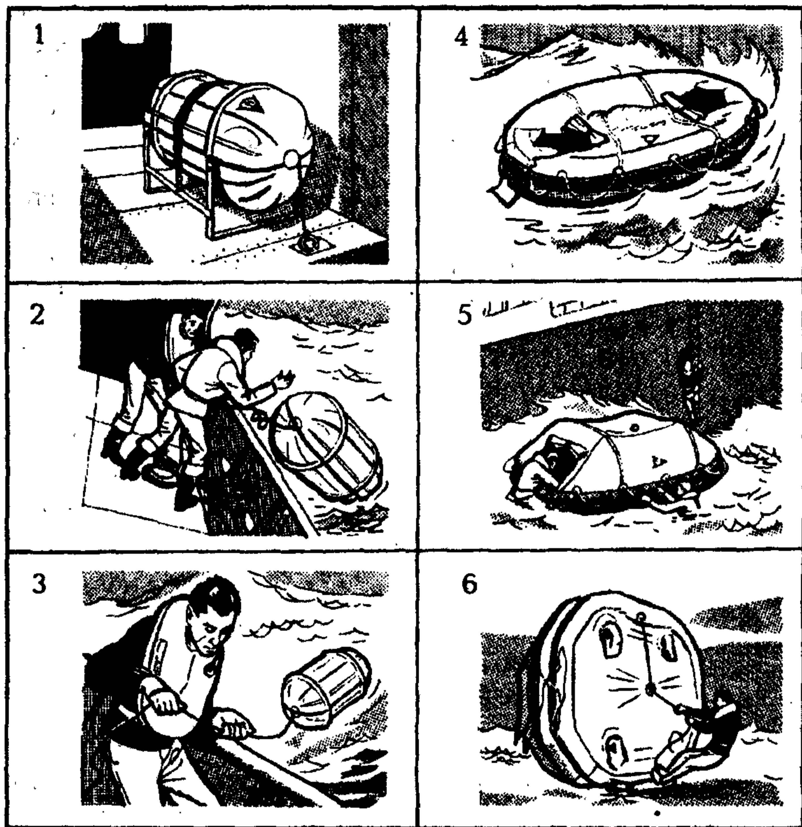
Рис. 23. Оставление судна на спасательном плоту:
