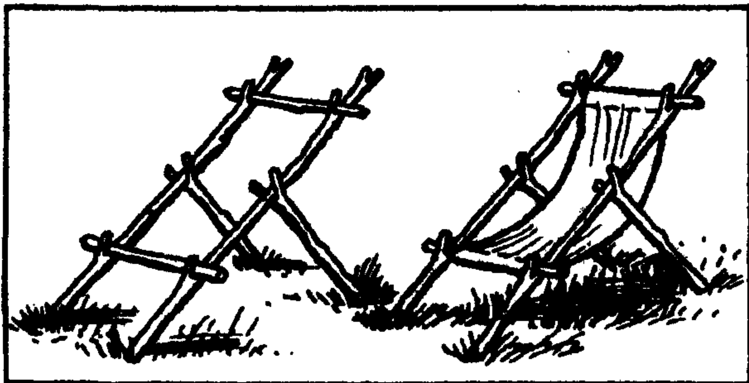
Рис. 61. Самодельный шезлонг.
