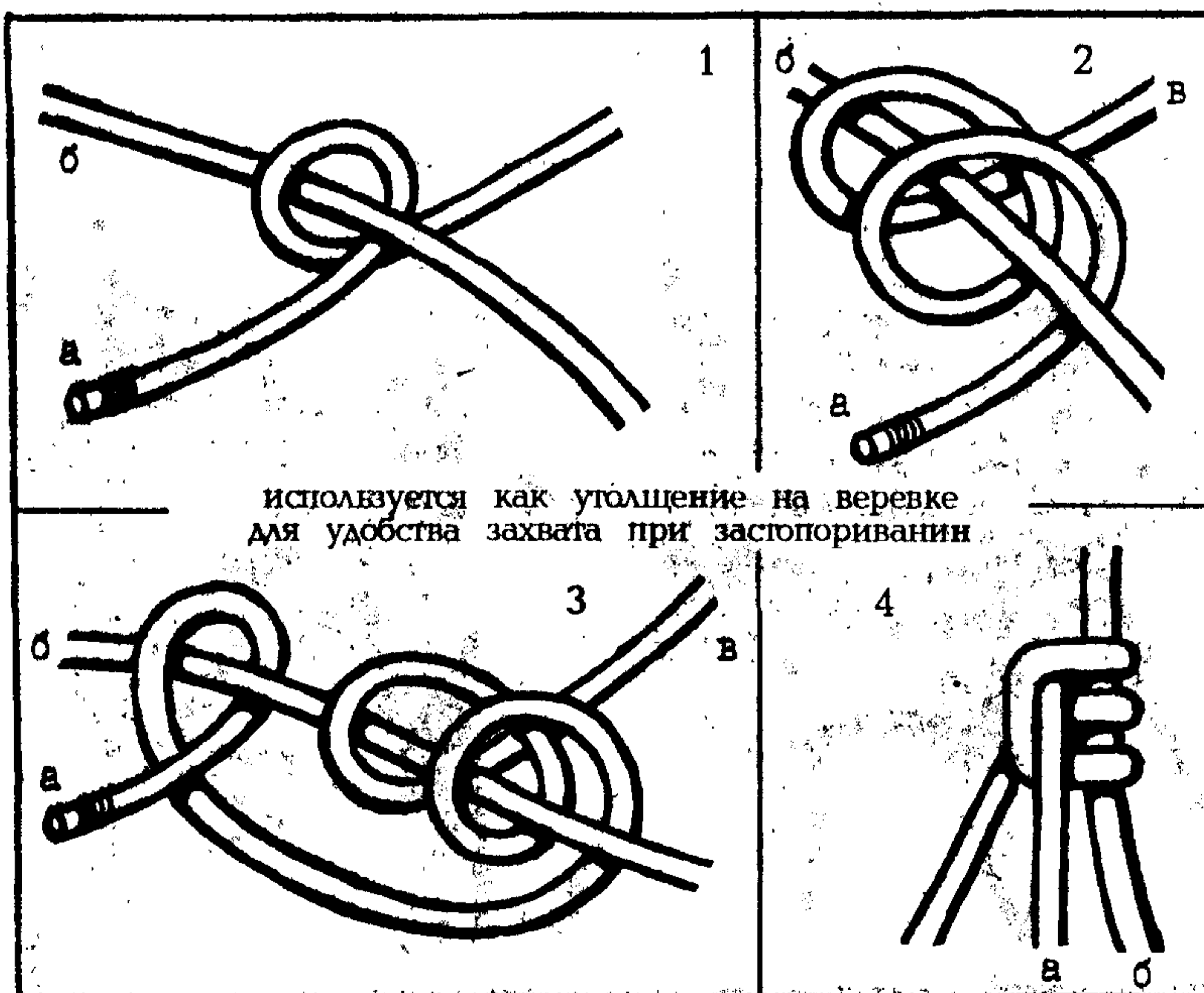
Рис. 218. Стопорный узел.
