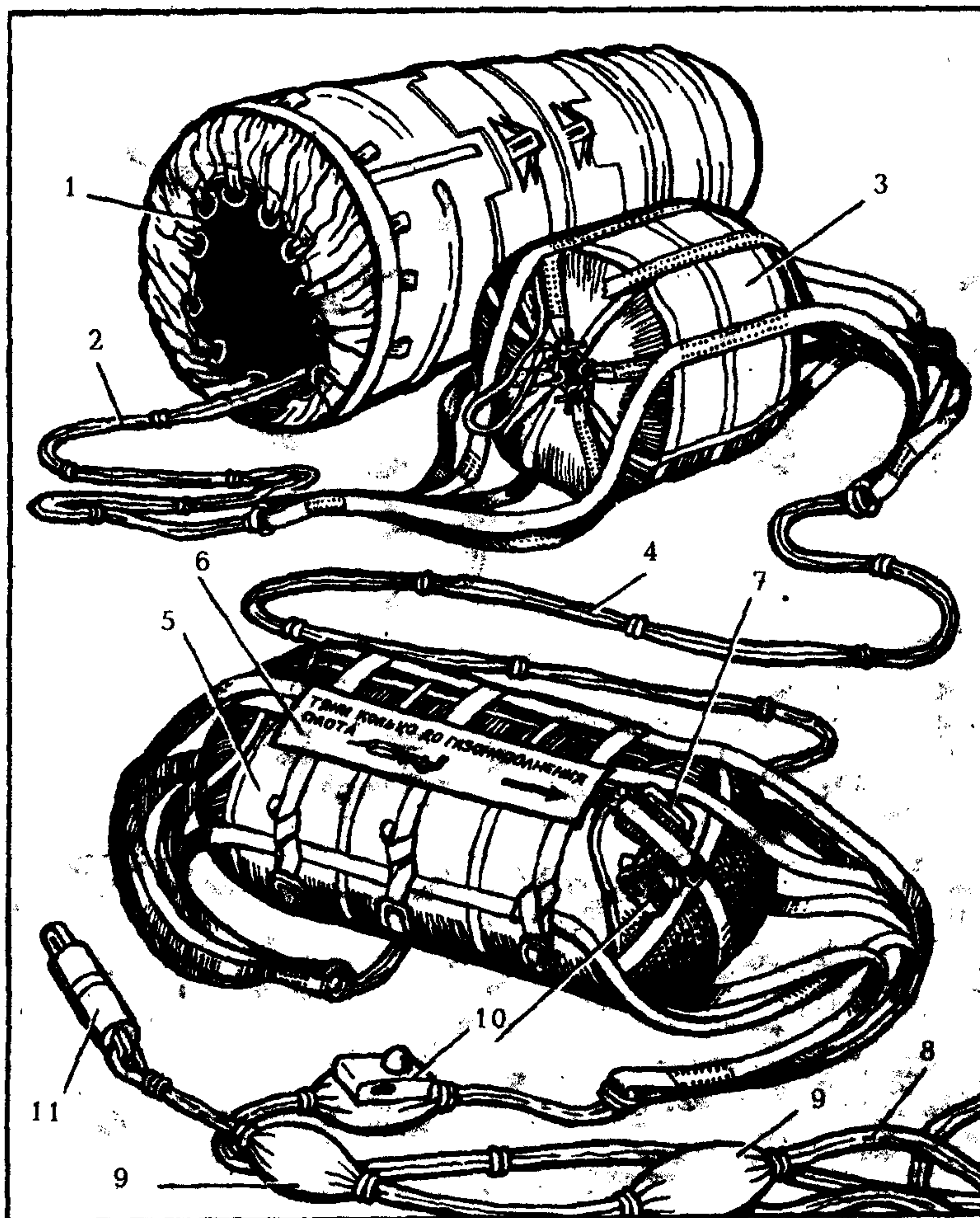
Рис. 259. Устройство спасательного контейнера КАС-150:
