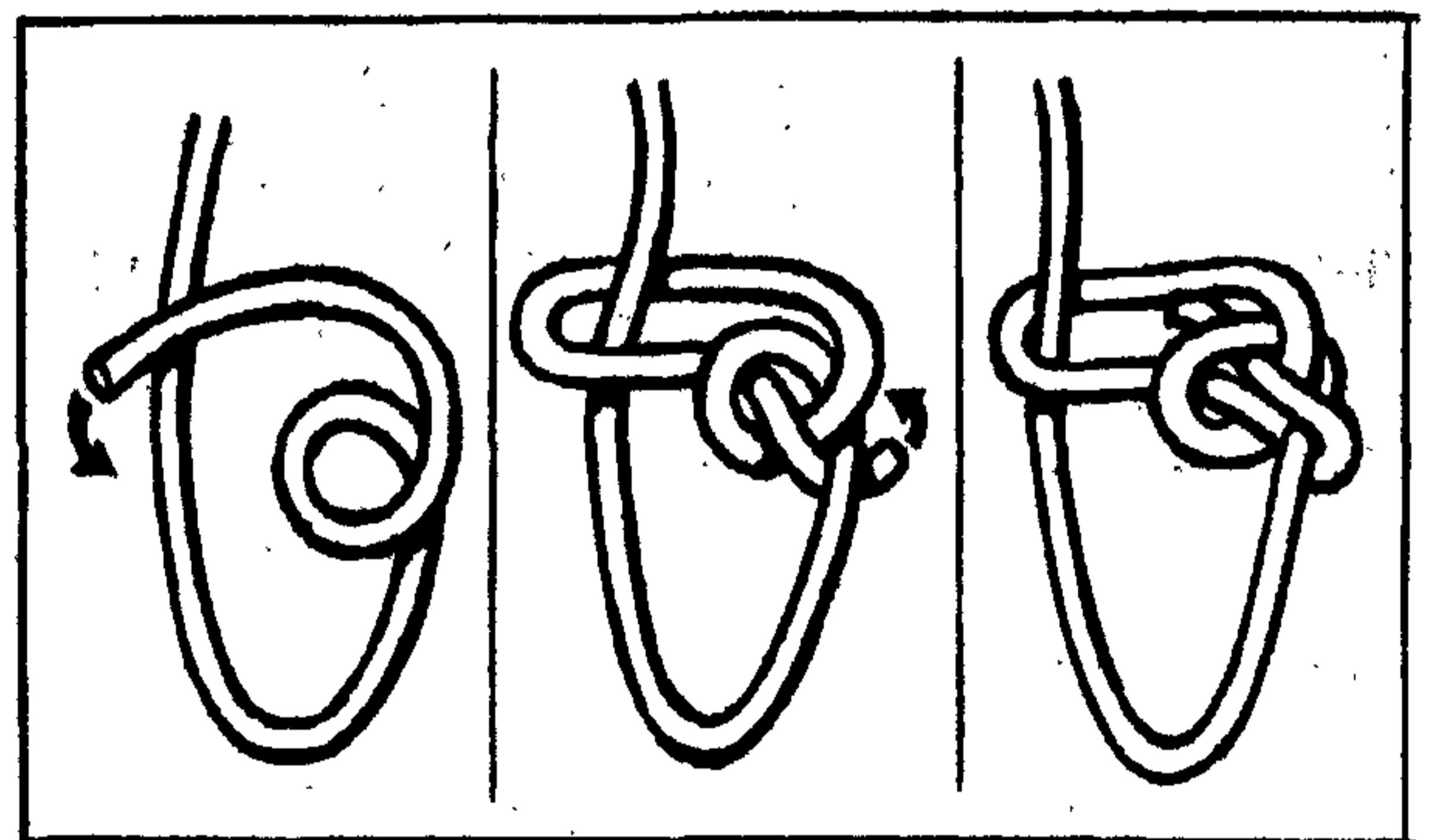
Рис. 219. Самозатягивающийся беседочный узел.
