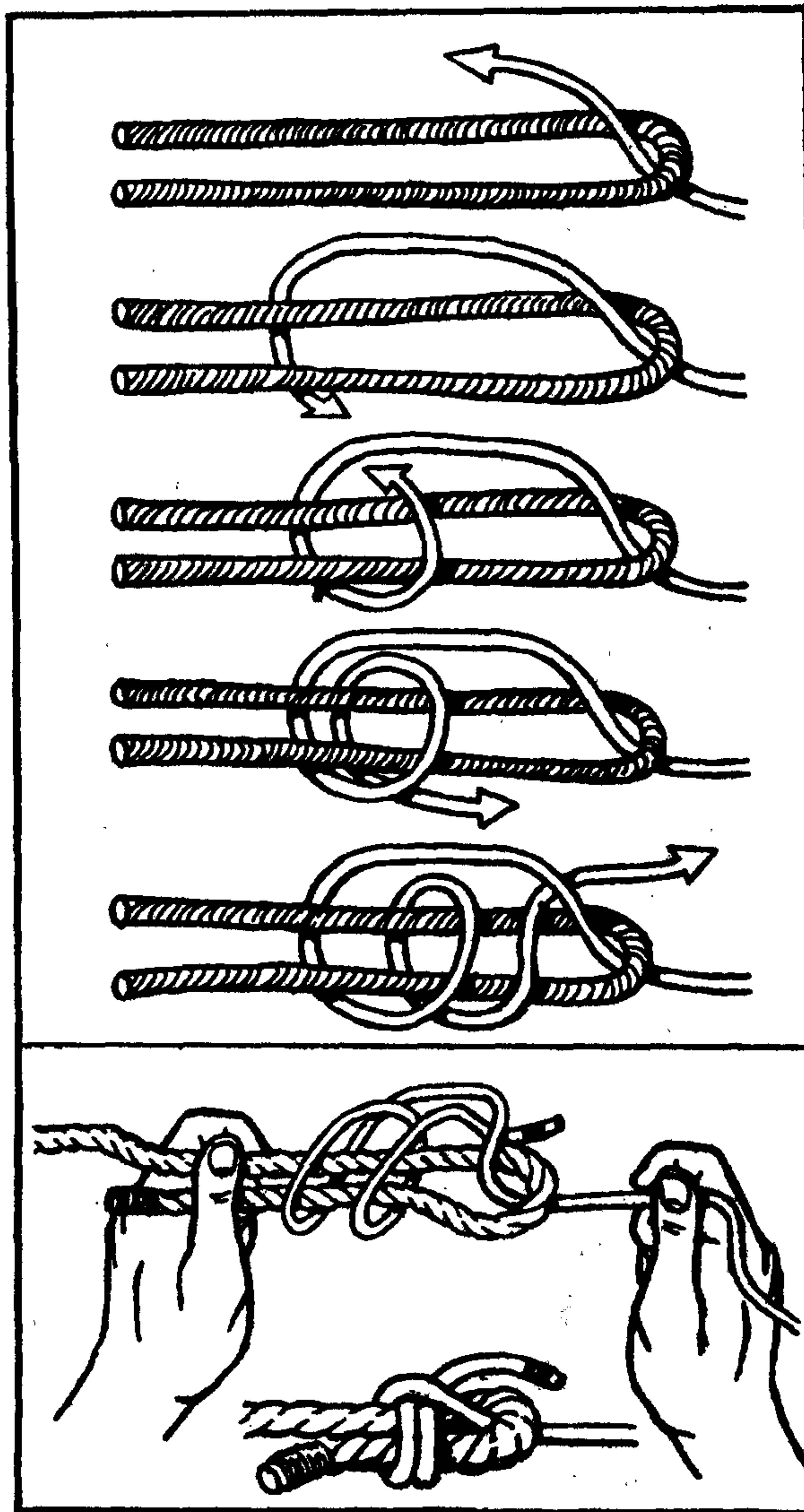
Рис. 212. Брамшкотовый узел.
