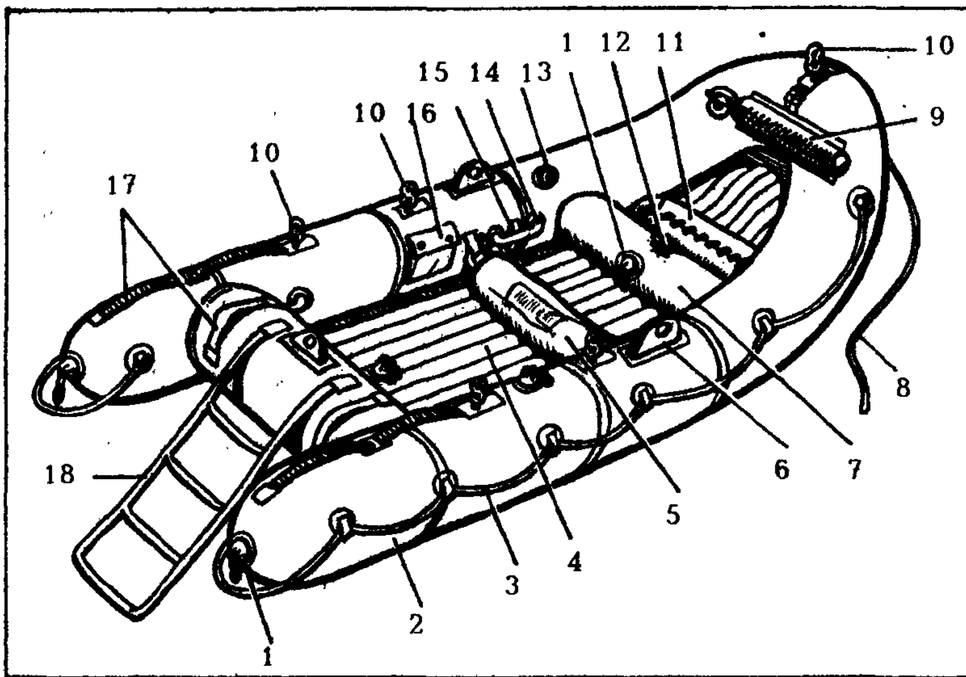
Рис. 279. Спасательная лодка ЛАС-5М-3:
