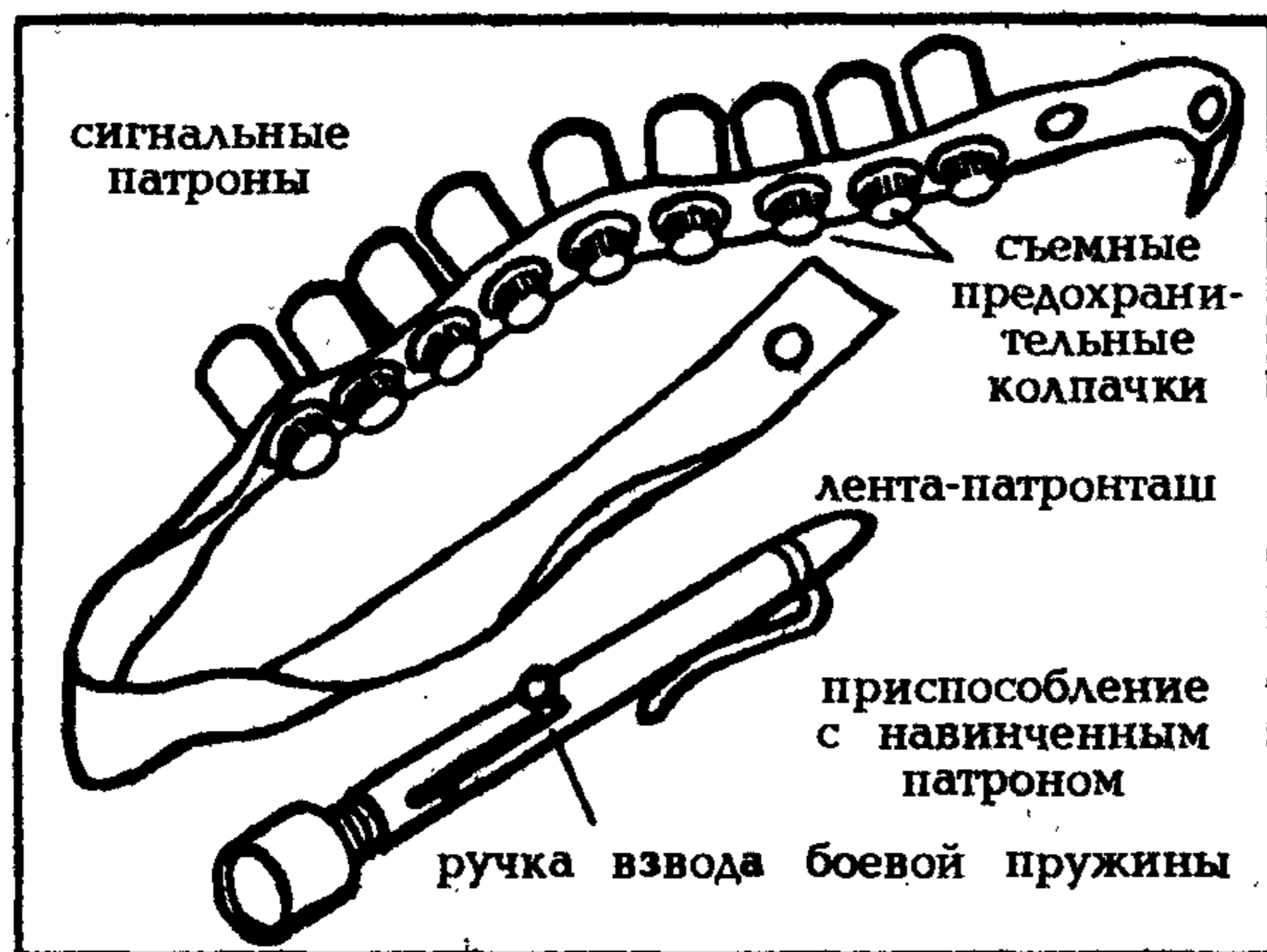
Рис. 267. 15-мм сигнальные патроны с приспособлением для отстрела.
