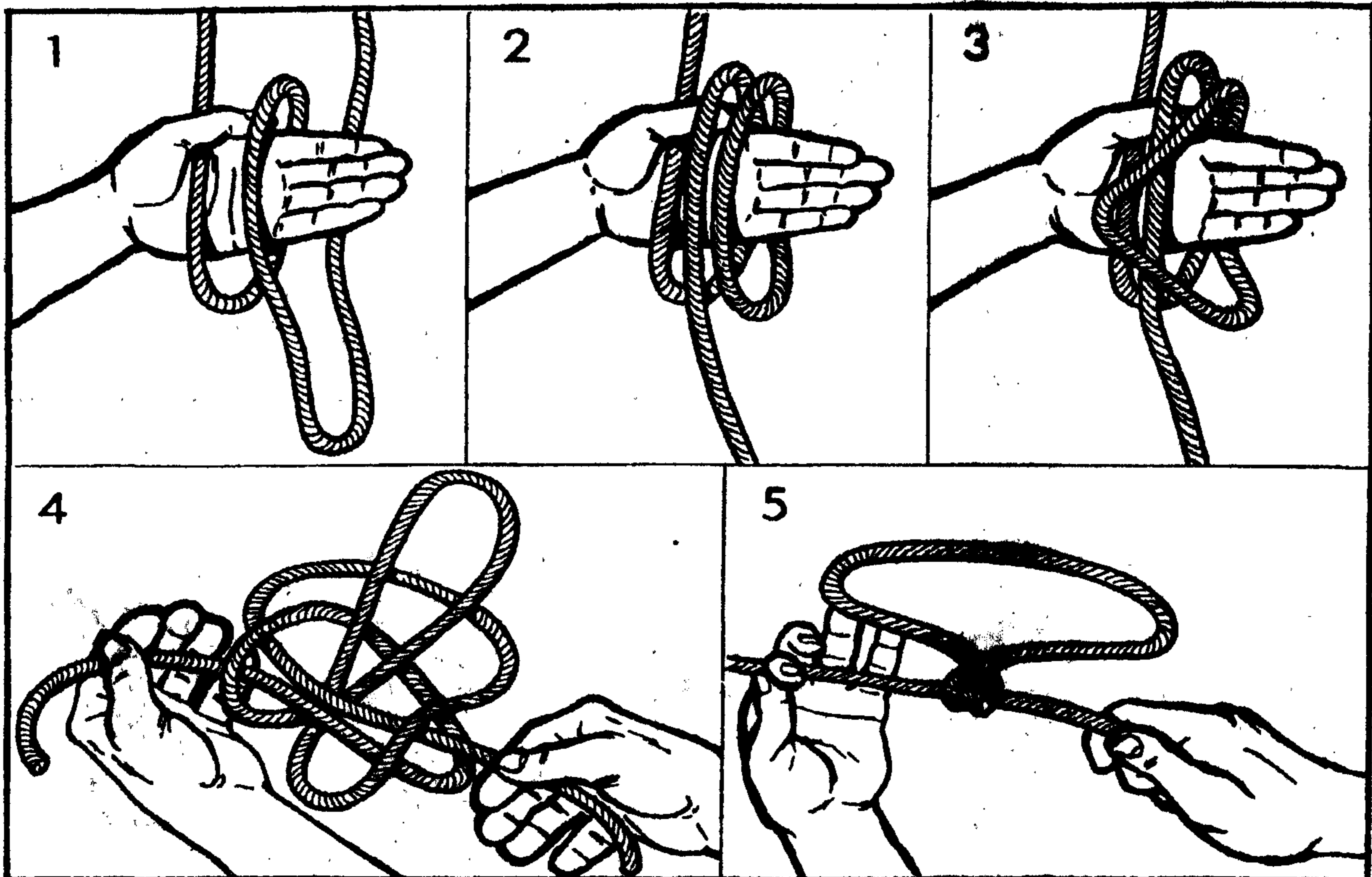
Рис. 209. Узел "бабочкой".
