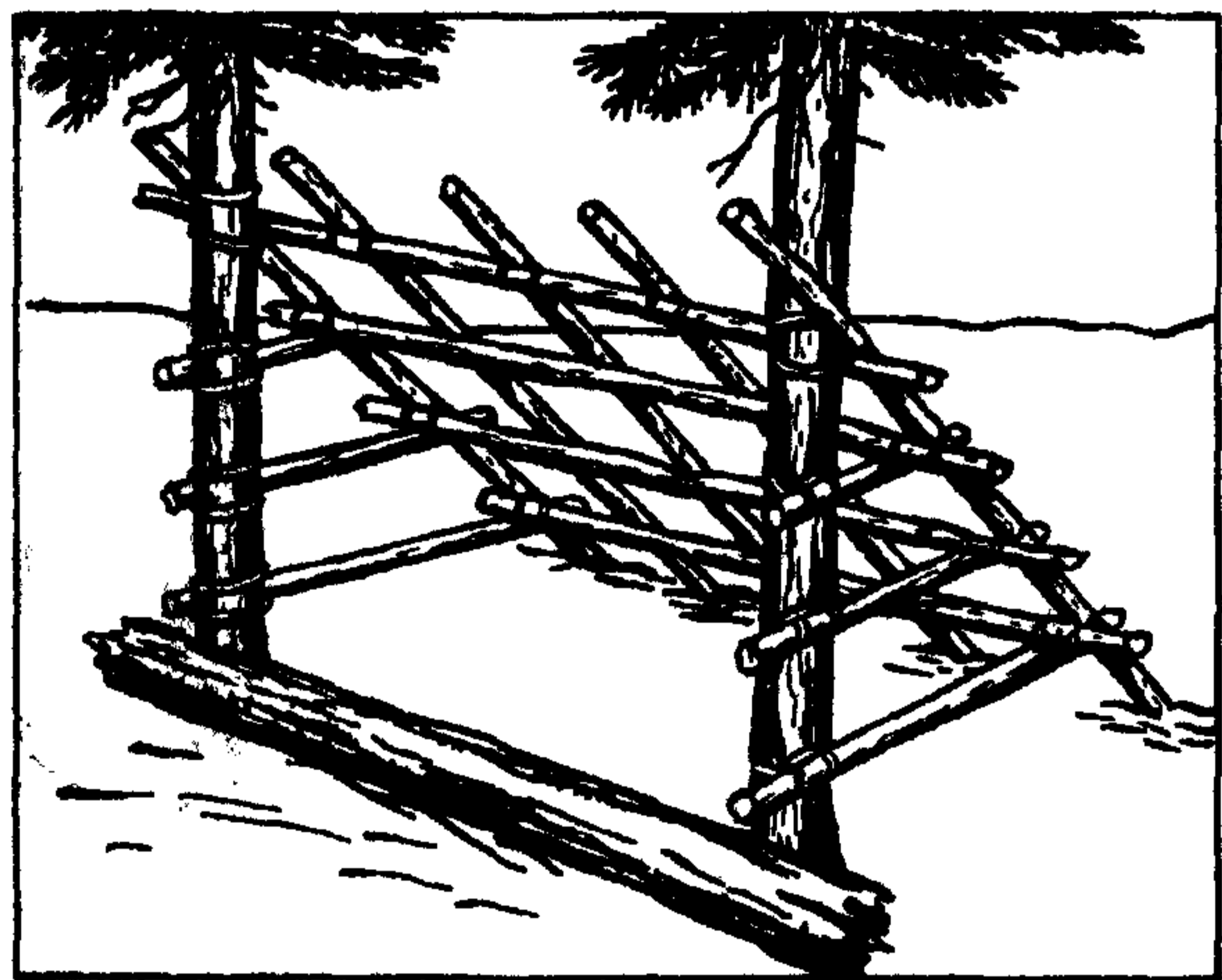
Рис. 43. Навес с односкатной крышей (каркас).
