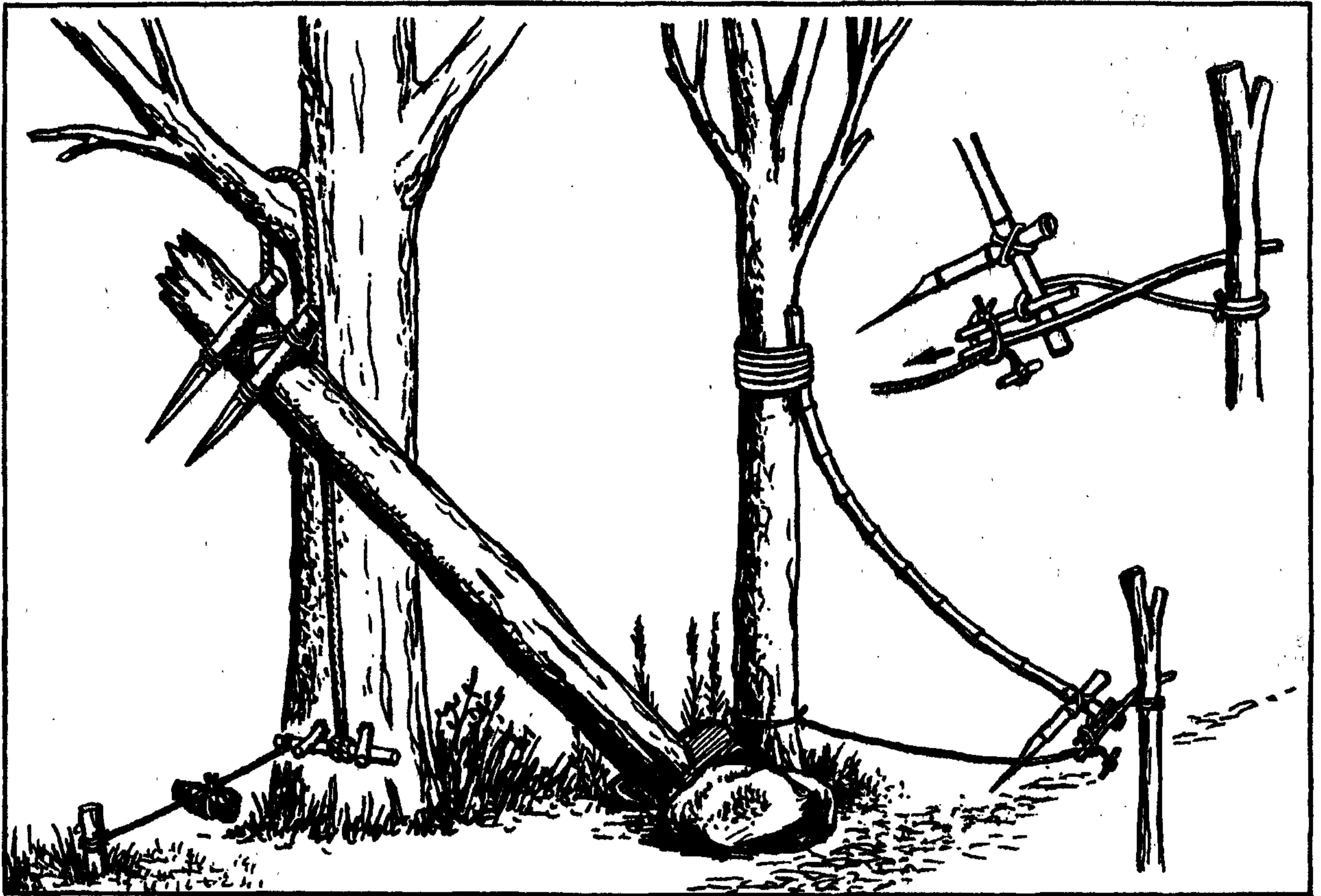
Рис. 108. Пронзающие ловушки.
