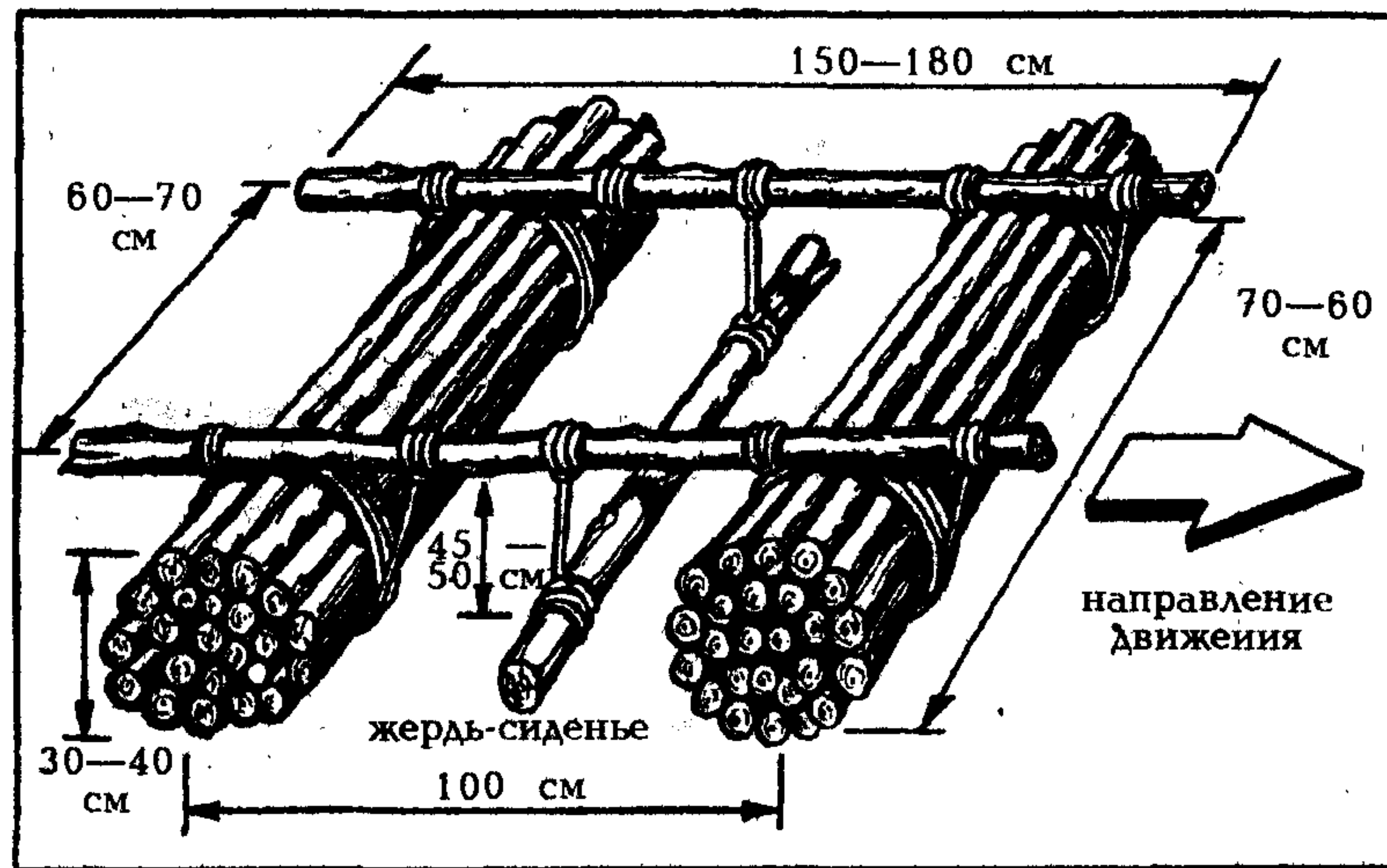
Рис. 176. Плот из жердевых связок.
