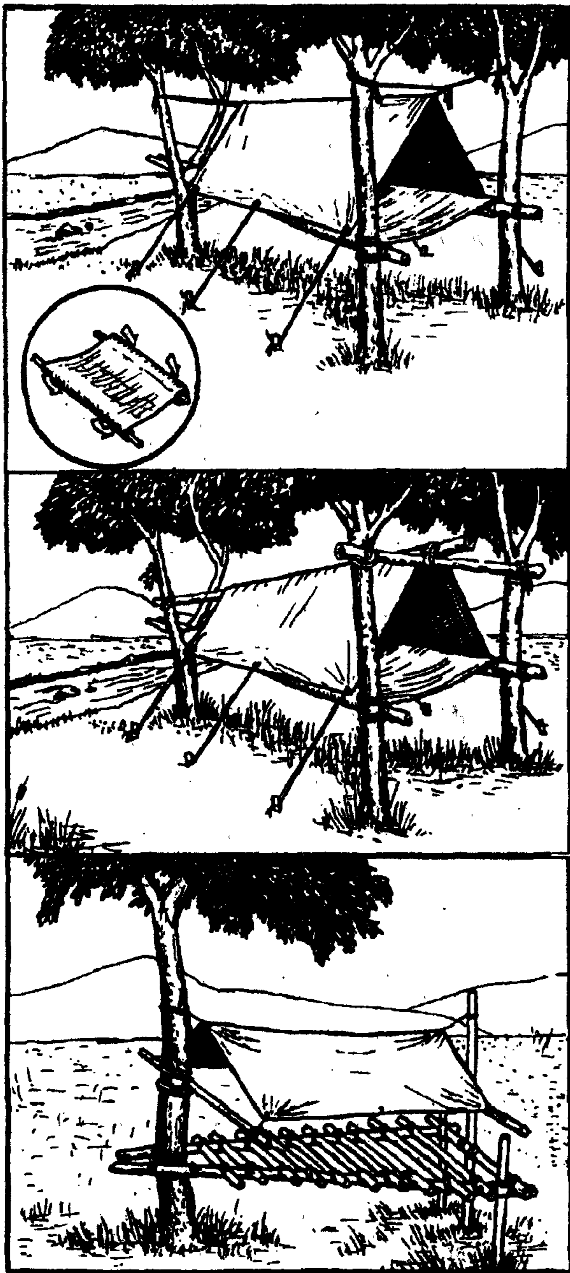
Рис. 46. Приподнятые укрытия.
