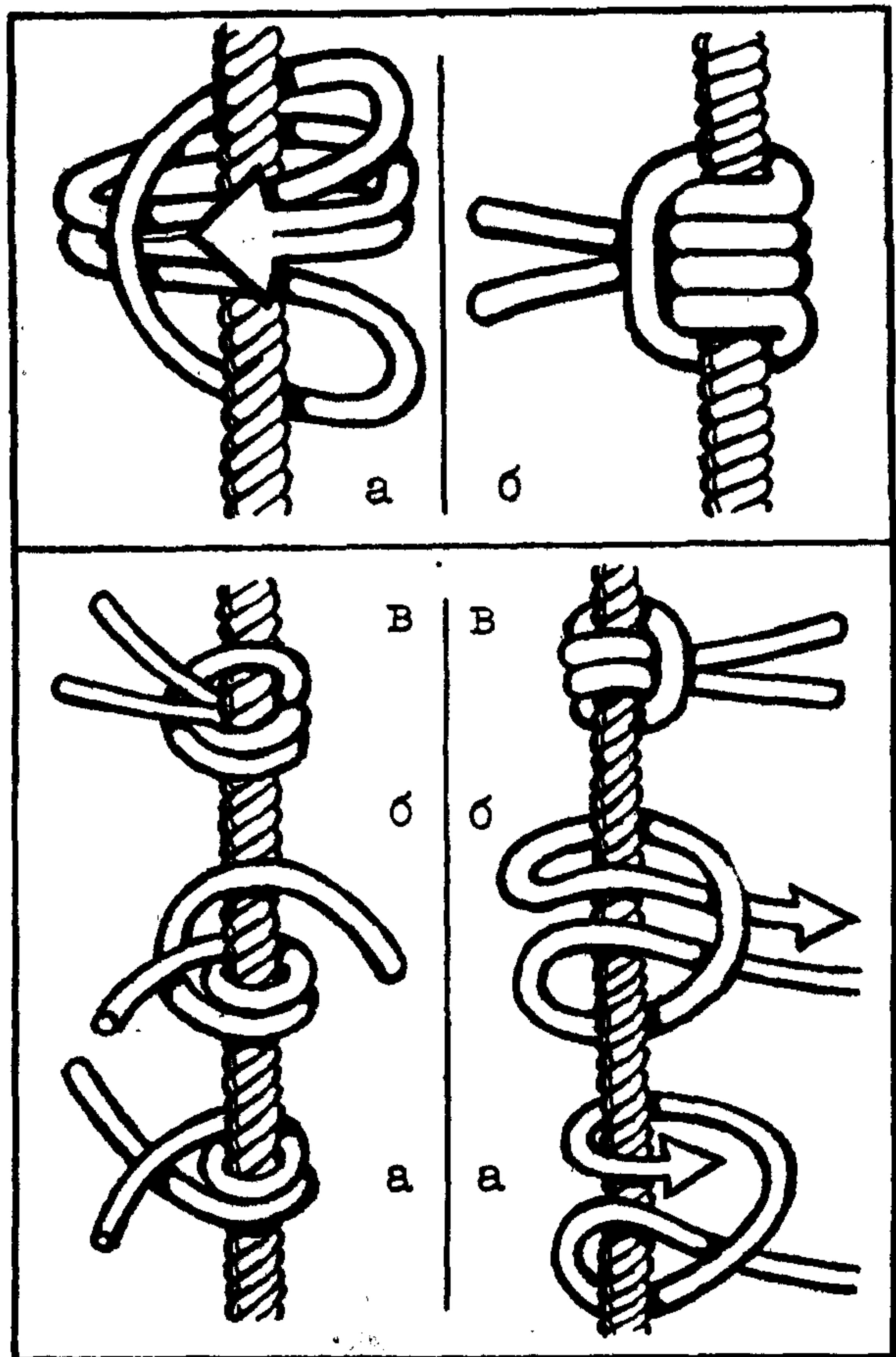
Рис. 210. Схватывающие узлы.
