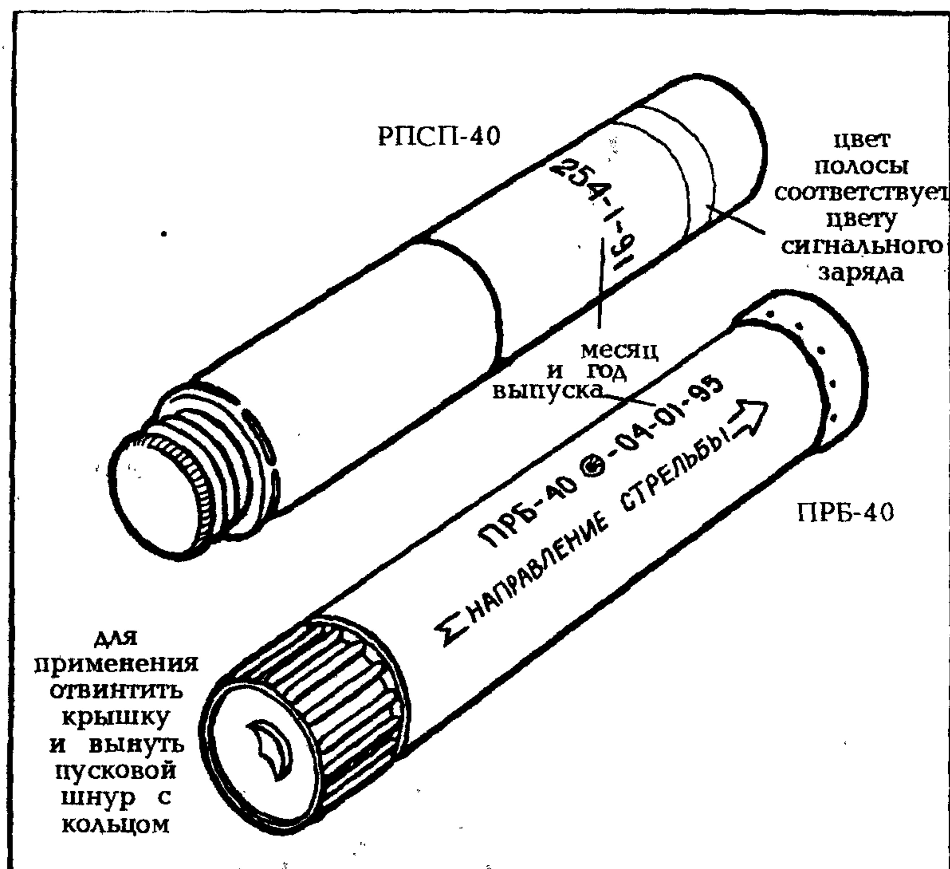
Рис. 271. Сигнальные реактивные патроны с парашютом.
