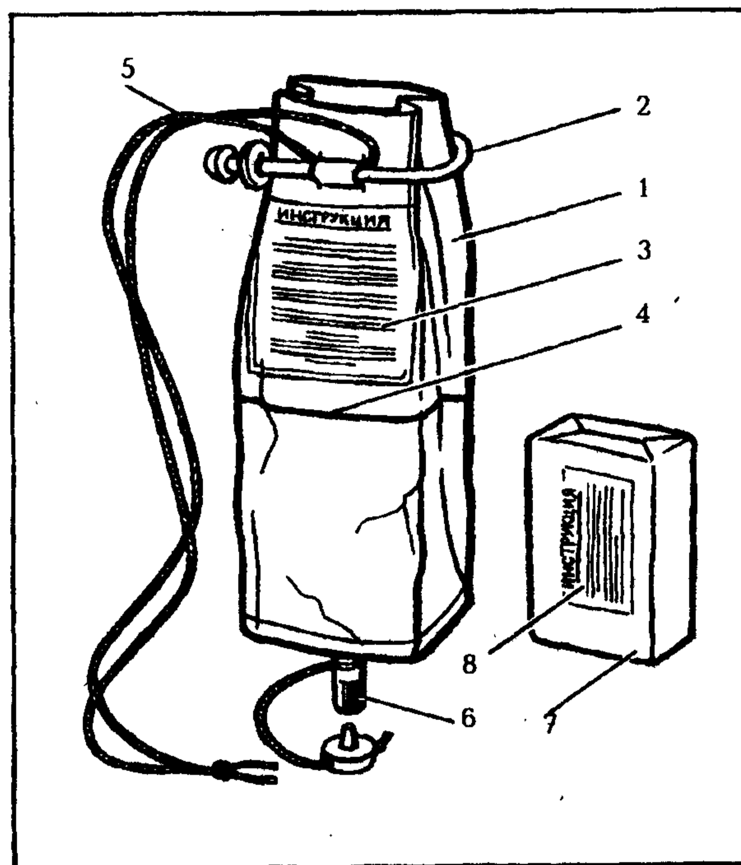
Рис. 255. Химический опреснитель морской воды ХО-2:
