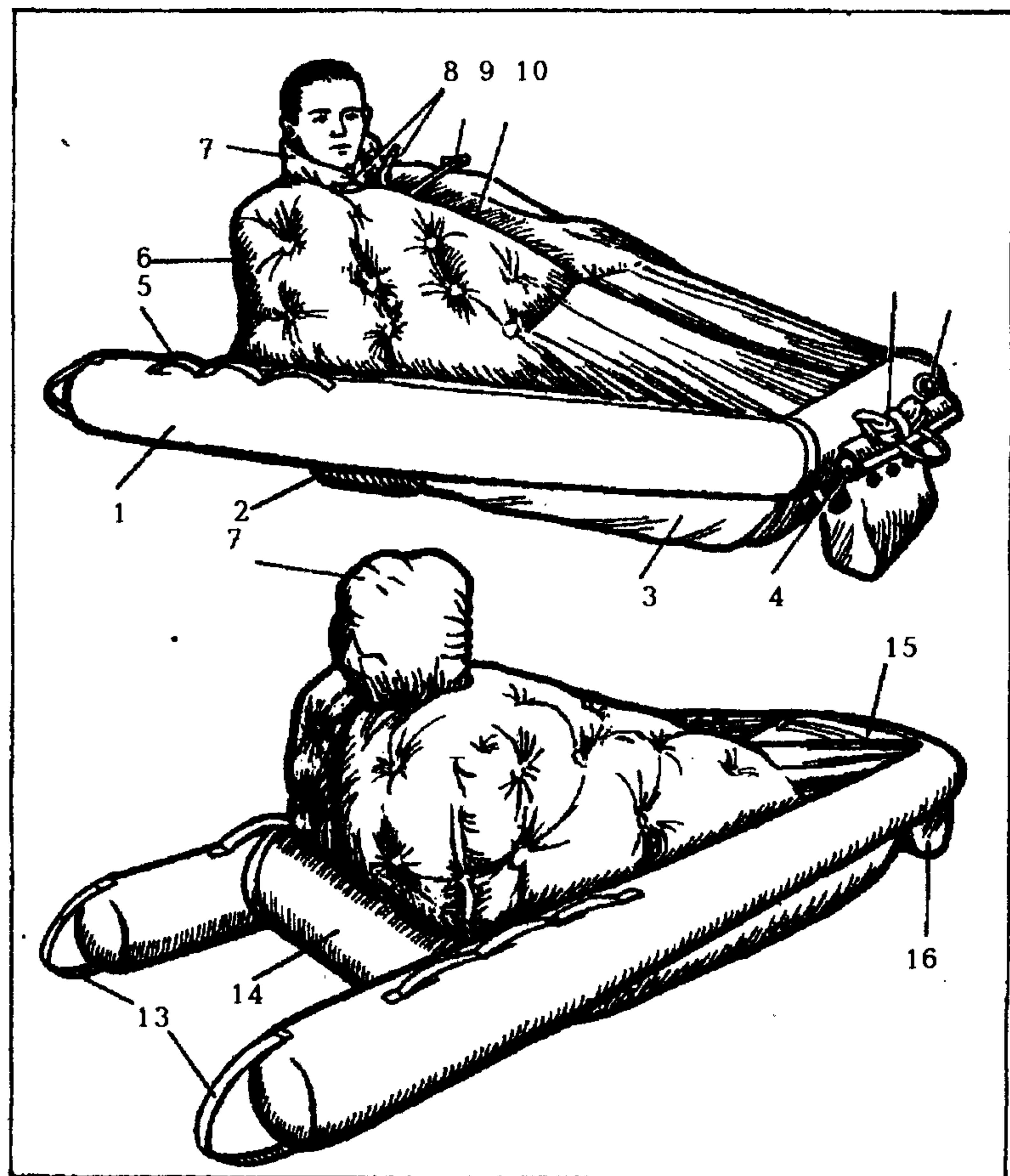
Рис. 278. Спасательный плот ПСН-1:
