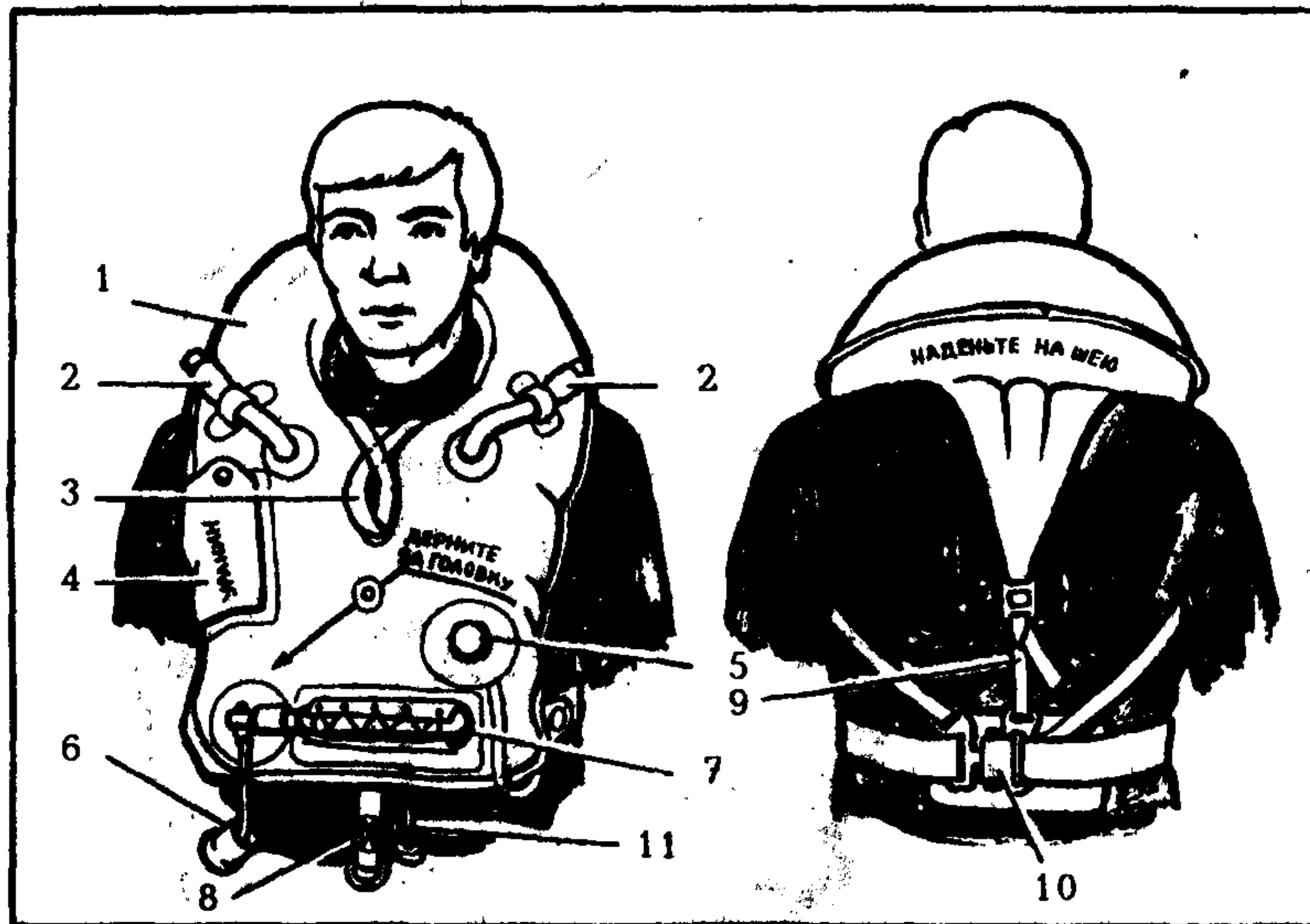
Рис. 273. Спасательный жилет АСЖ-58 (в надутом состоянии):
