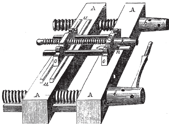
Рис. 5-й. Обрѣзной прессъ съ наложеннымъ на него гобелемъ. АААА—станокъ; в в —винты; оо —гобель; и и —желобокъ, по которому ходитъ гобель; н —рѣзакъ гобеля; к —винтъ, управляющій рѣзакомъ.
