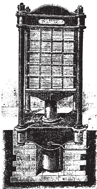
Рис. 43-й. Гидравлическій прессъ съ зажатými въ немъ, между дощечками, пачками печатныхъ листовъ.
