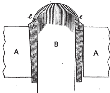
Рис. 86-й. Книга (В) зажата въ прессъ (А А) между двумя дощечками ( o и o ), скошенными не только у верхнихъ краевъ ( e и e ), но также и по плоскости: для того, чтобы давленіе сосредоточивалось главн. образомъ именно у фальцовъ ( e и e ).
