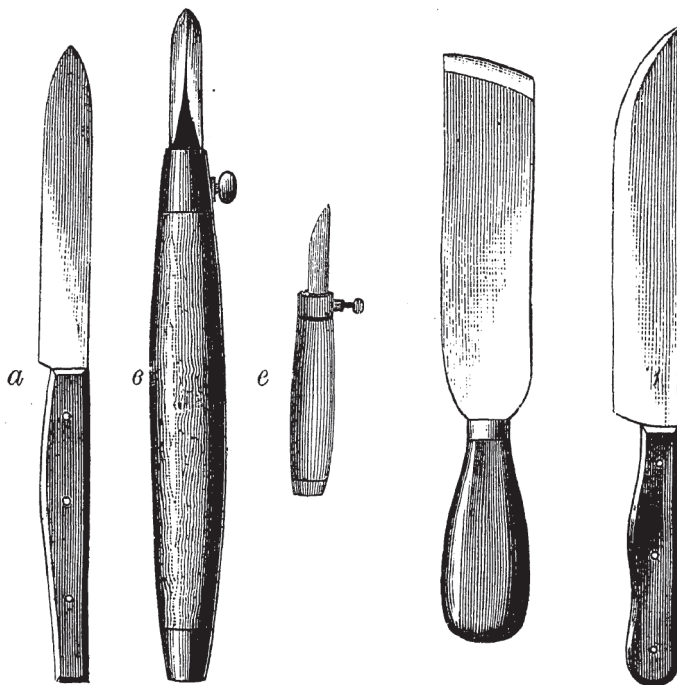
Рис. 19-й. a —нож для рѣзанія бумаги; b и c —ножи для рѣзанія картона (съ перемѣнн. клинкомъ).
