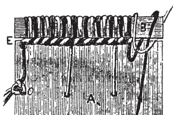
Рис. 118-й. Плетение простого капитала въ двѣ нитки почти окончено. Значеніе буквъ то-же, что на рис. 117-мъ. Такое-же и увеличеніе.
