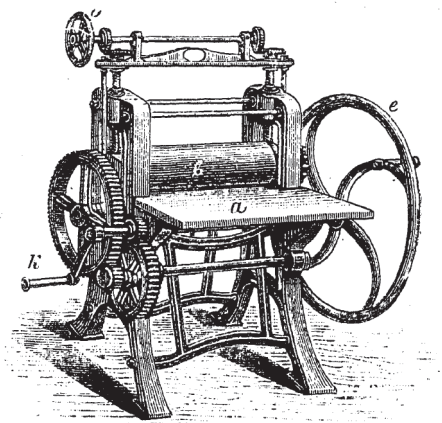
Рис. 40-й. Сатинировавальная машина.
