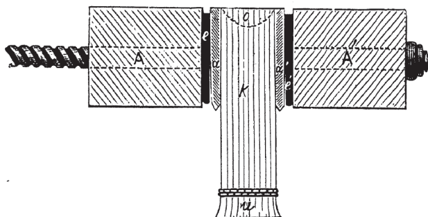
Рис. 109-й. Зажимание книги для золочения передка: А А' — пресс; к — книга, и — корешок, о — передок; а и а' — скошенные по плоскости шпальты; е и е' — нескошенные (плоския) шпальты.
