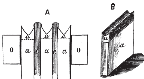
Рис. 87-й. Въ А двѣ книги (e, e), зажаты въ прессѣ (o o) между тремя дощечками (a, a, a) съ двойными острыми верхними краями (u, u, u); въ В одна такая дощечка.
