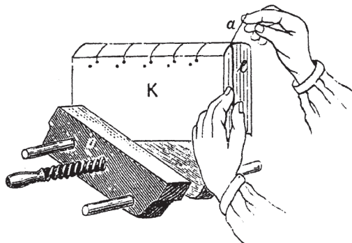
Рис. 116-й. Зажиманіе книги въ прессъ для плетенія капітала: к —книга; о —прессъ; е —обрѣзь головки или хвоста книги; а —двѣ нитки, при помощи которыхъ плетется капіталъ. На картонѣ видны два ряда дырочекъ, сквозь которыя продѣты шнуры, прикрѣпляющіе картонъ къ книгѣ (см. ниже — третій способъ прикрѣденія картоновъ къ книгѣ).
