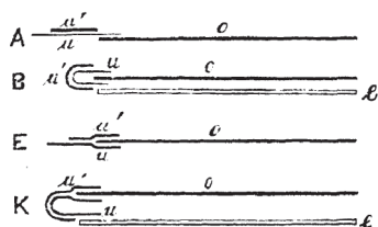
Рис. 60-й. Приклеиваніе рисунковъ ( o ) на коленкоров. фальцахъ съ бумажною подклейкою послѣднихъ: u — полоска коленкора; u' — полоска бумаги; e — тетралин.
