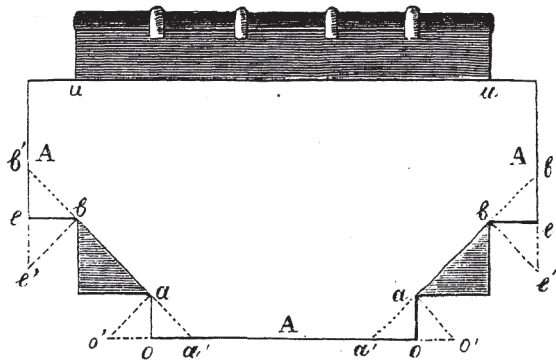
Рис. 140-й. Выкройка коленкора или бумаги при полужокожанномъ переплетѣ. A, A и A —запасы коленкора или бумаги для заворотовъ на внутреннюю сторону картона; u u — линія края выкройки вдоль корешка. Относительныя значенія остальныхъ буквъ см. текстъ.
