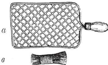
Рис. 16-й. a —сѣтка для крапленія обрѣзовъ; b —кисть къ ней.
