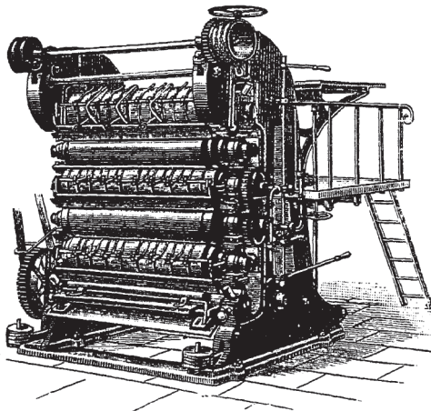
Рис. 42-й. Каландръ.
