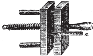
Рис. 6-й. Гобель; a —рѣзакъ.
