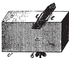
Рис. 90-й. Правая колодка гобеля, повернутая низомъ ( о ) вверхъ, а верхомъ ( о' ) внизъ; п —рѣзакъ; а —проходящій внутри колодки болтикъ, обозначенный точечн. линіями; е и е —лапки болтика; в —гайка, навинчиваемая на верхній конецъ болтика.
