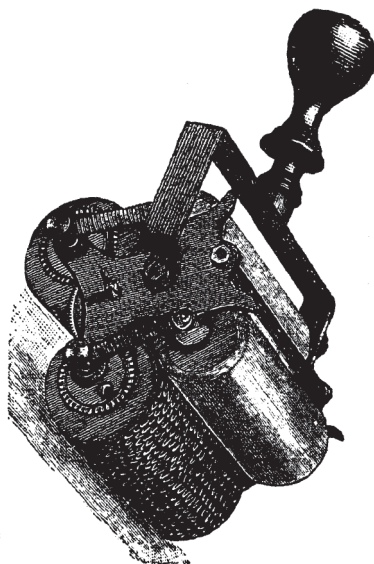
Рис. 39-й. Апаратъ для мраморирования обрѣзовъ сь 2 рисо- вальными валиками.
