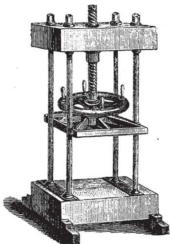
Рис. 36-й. Паковальный пресс большей величины, также же- лезный, но сь деревянн. нижн. и верхн. досками.
