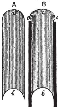
Рис. 79-й. А: корешок (а) книги округлен послѣ обрѣзки передка (б), вогнутость котораго вполне соотвѣтствует выпуклости корешка. В: та-же книга зажата между двумя дощечками въ прессѣ; у е и е начинаютъ, отъ давленія, образовываться фальцы.
