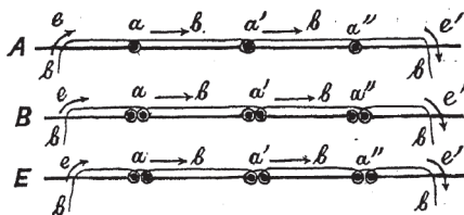
Рис. 78-й. Ведение нитки при шиваніи на шнурахъ безъ пропилки корешка—швомъ иголкою назадъ . А—шиваніе на оди- ночныхъ шнурахъ; В и Е—шиваніе на двойныхъ шнурахъ.
