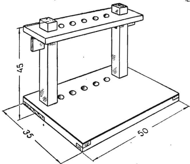
Рис. 2. Общий вид станка для шивания.
