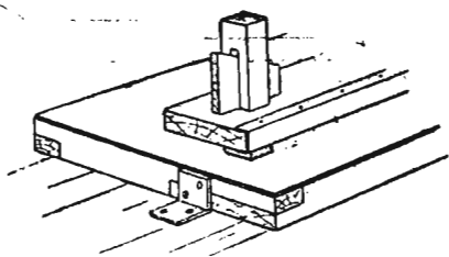
Рис. 12. Прикрепление зажима для обрезки к столу или верстаку.
