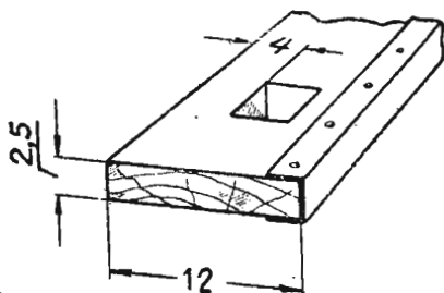
Рис. 11. Кромка доски, обитая жстью.
