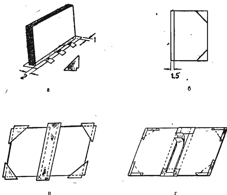
Рис. 23. Подготовка картонного переплета книги.
