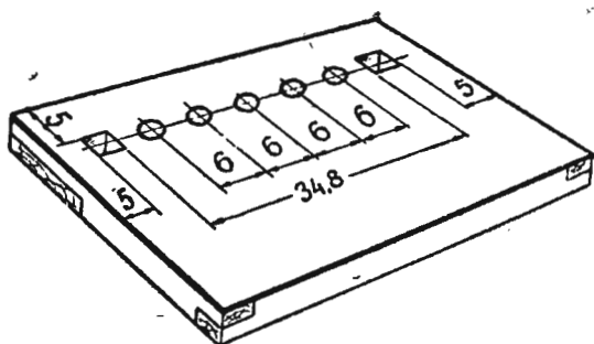
Рис. 5. Площадка станка.
