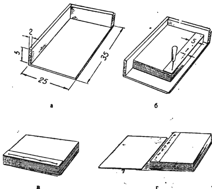
— Рис. 24. Переплетение книжек из одинарных листов.
