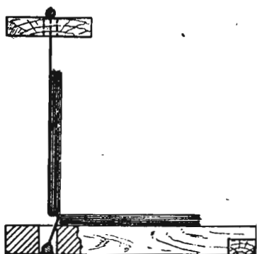
Рис. 25. Положение ремонтруемой книги, вновь пришиваемой к тесемкам.
