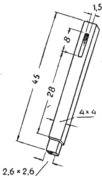
Рис. 4. Вертикальный брусок. просверлите коловоротом
