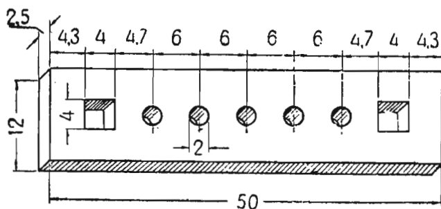
Рис. 6. Верхняя доска станка.
