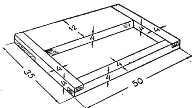
Рис. 3. Рамка станка.
