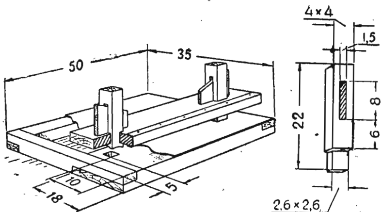
Рис. 10. Зажим для обрезки.
