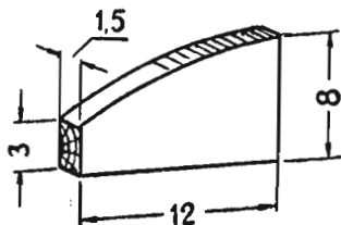
Рис. 8. Клинышек.
