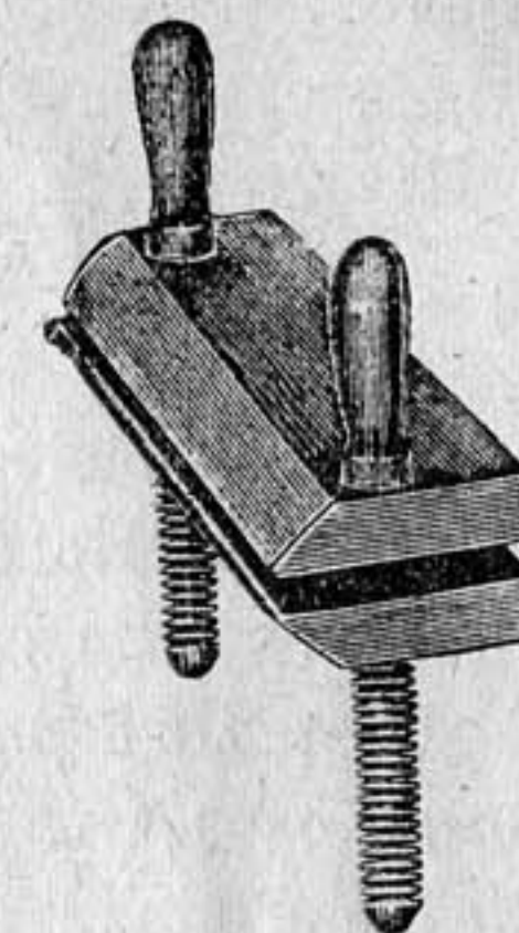
Прессъ для золоч.
