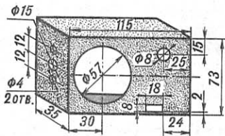
Рис. 4. Корпус.
