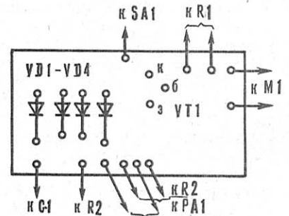
Рис. 6. Печатная плата со схемой расположения элементов (вариант II).
