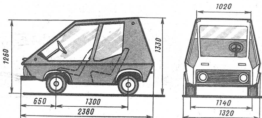
Микроавтомобиль КЮА.
