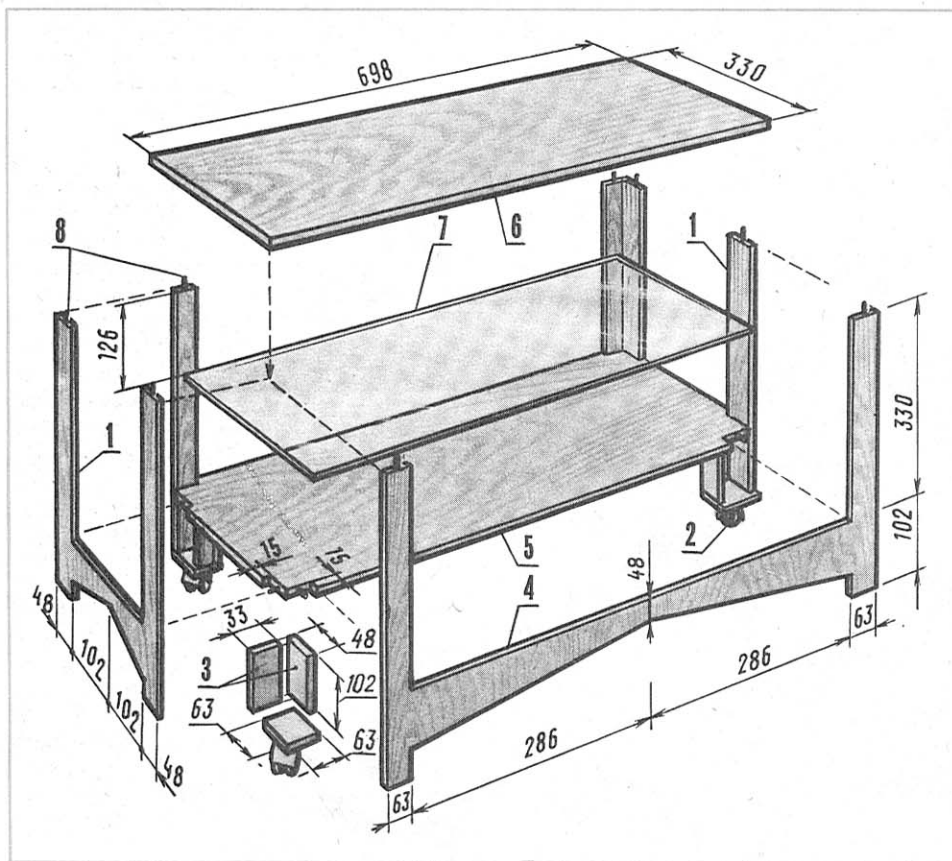
Колесный столик:
