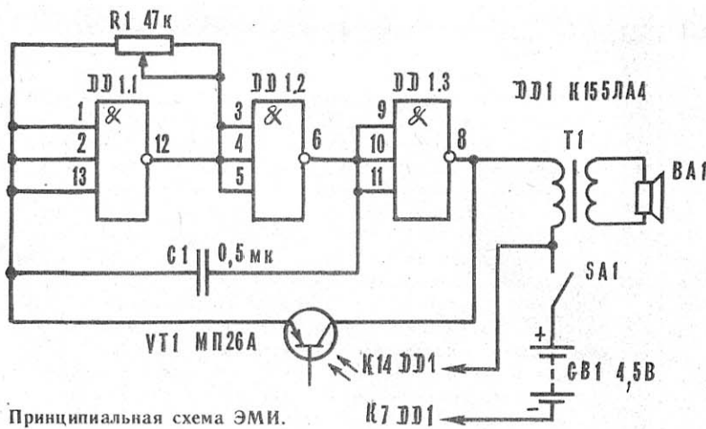
Принципиальная схема ЭМИ.
