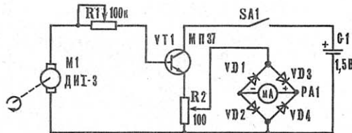
Рис. 2. Схема тахометра для электродвигателей (VD1—VD4 Д9А).
