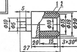
Рис. 5. Переходник: 1 — вставка, 2 — резиновая втулка.
