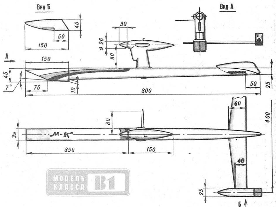
Кордовая скоростная модель аэроглицсера с двигателем внутреннего сгорания рабочим объемом 2,5 см 3 .
