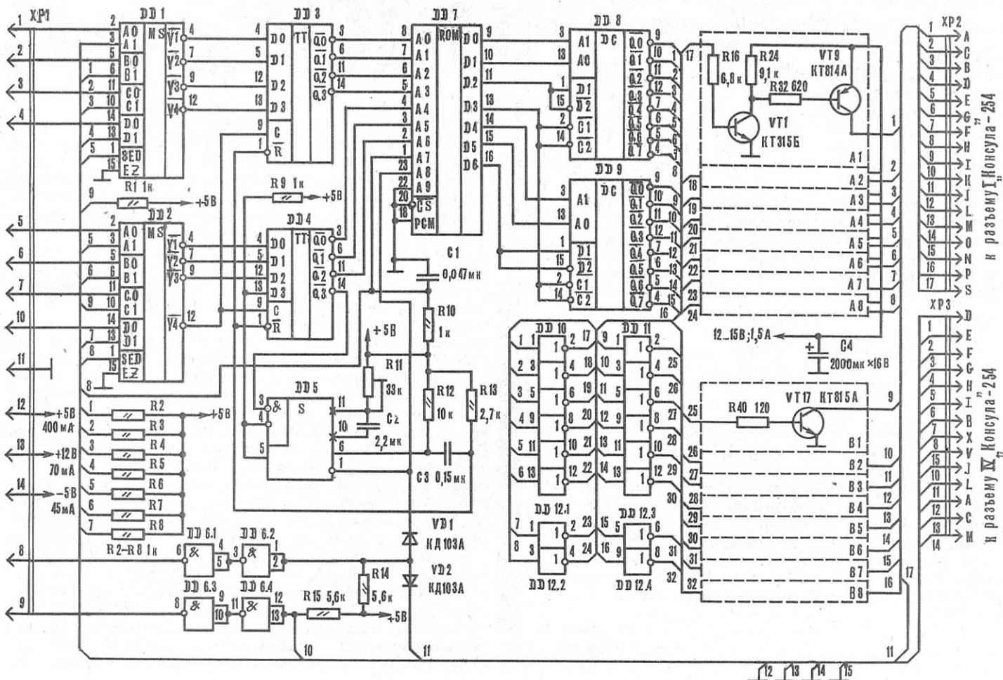
Р и с. 2. Принципиальная схема контроллера: DD1, DD2 K555КП14, DD3, DD4 K155ТМ8, DD5 K155АГ1, DD6 K155ЛА3, DD7 K573РФ1, DD8, DD9 K155ИД4, DD10 — DD12 K155ЛН1.
