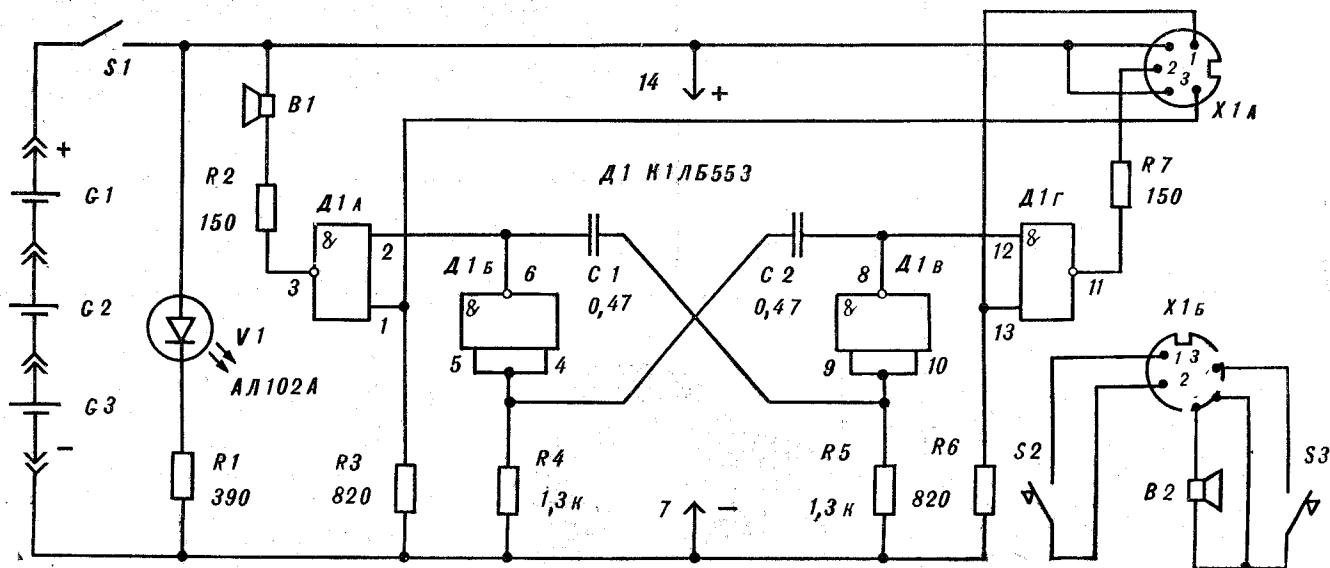
Рис. 1. Принципиальная схема тренажера.
