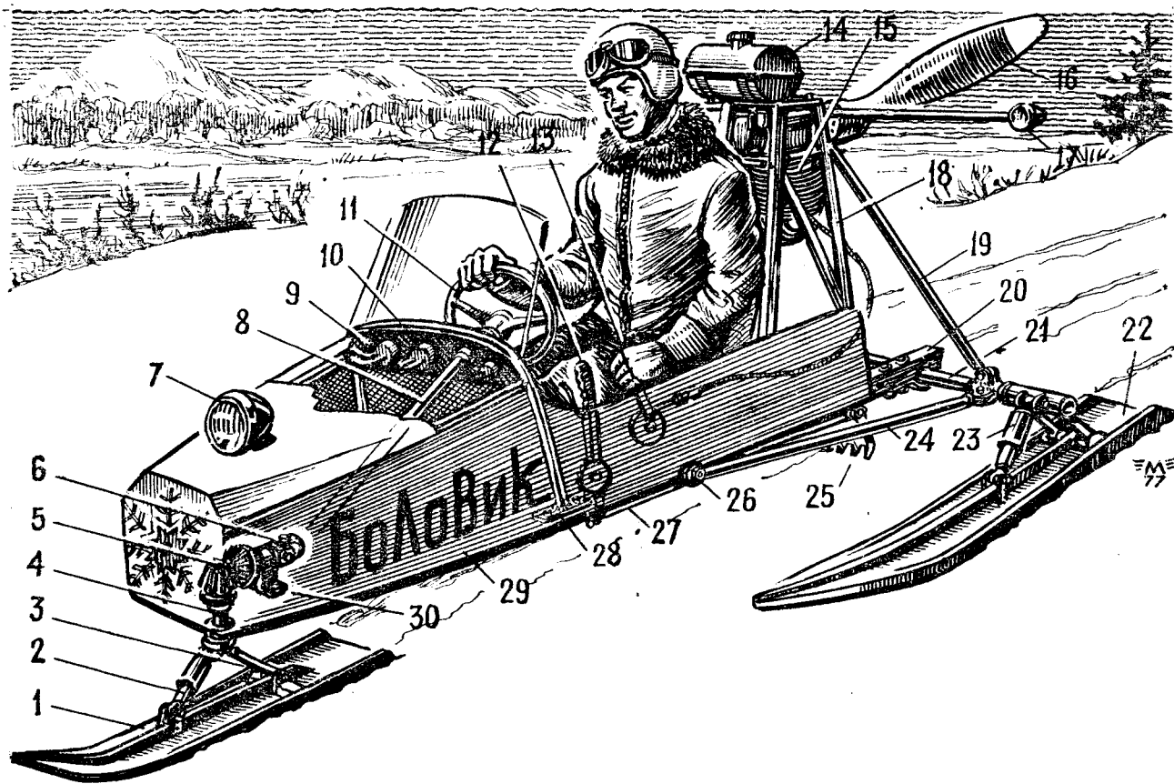
Рис. 1. Общий вид аэросаней:
