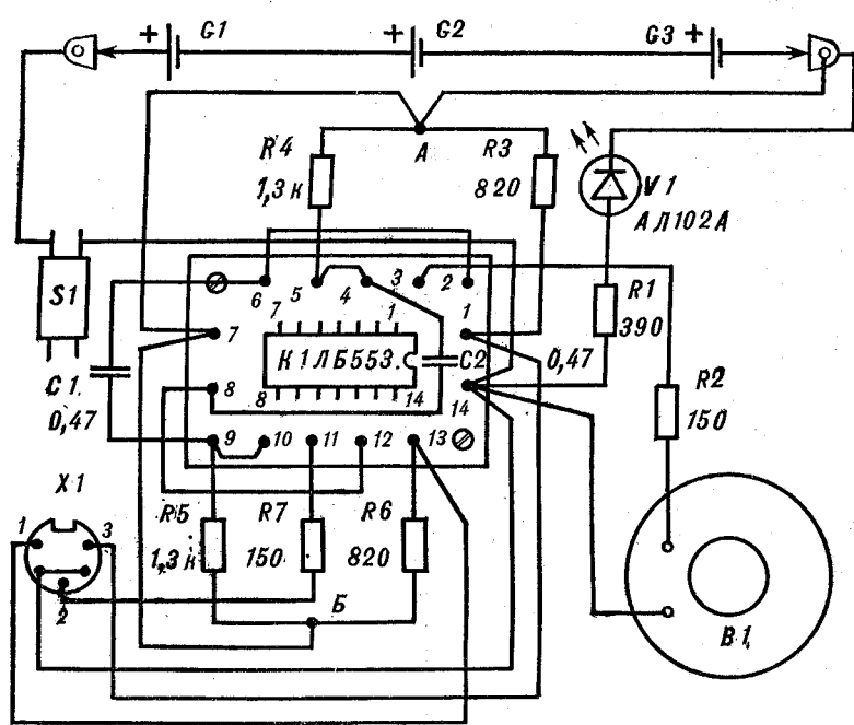
Рис. 2. Монтажная схема тренажера.
