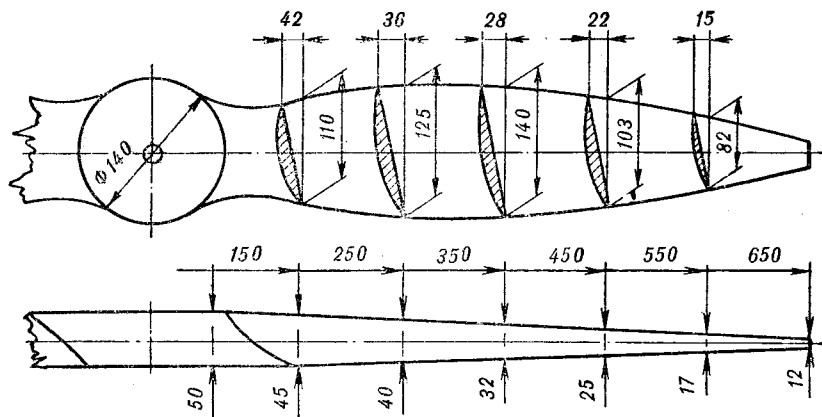
Рис. 3. Схема в двух проекциях: А — вид сбоку; Б — вид сверху.
