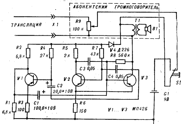
Рис. 1. Принципиальная схема звонка.
