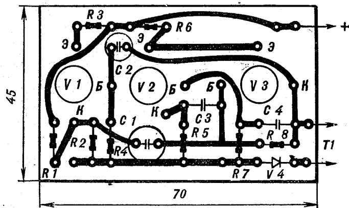
Рис. 2. Печатная плата звонка с расположением деталей.
