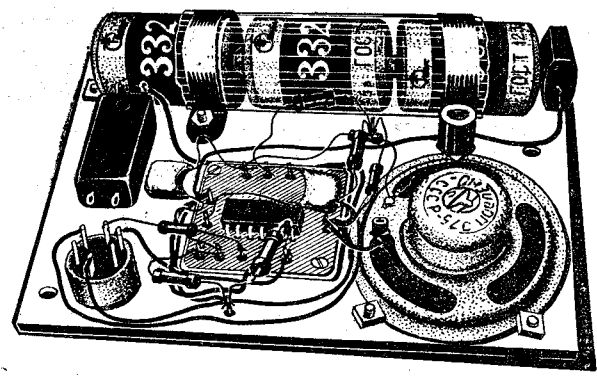
Рис. 4. Расположение элементов схемы на плате.
