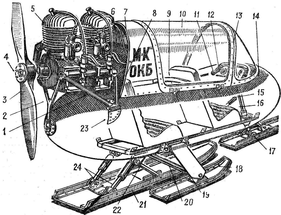
Рис. 1. Общая компоновка аэросаней:
