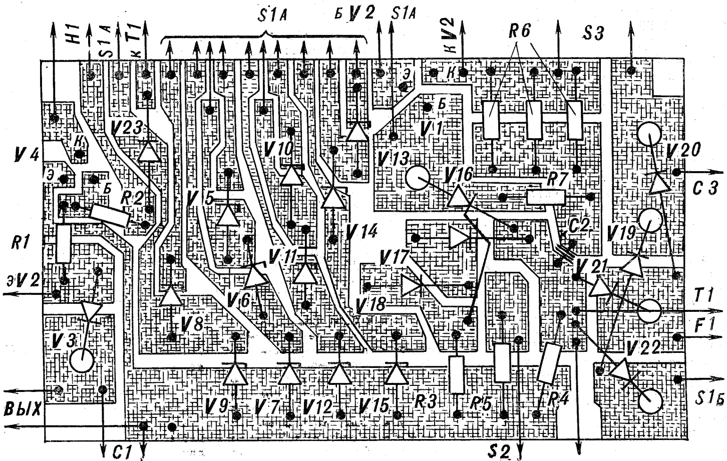
Рис. 2. Печатная плата с расположением деталей.
