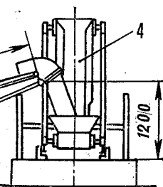
Рис. 3. Разгрузка вагона транспортером: 1 — ленточный транспортер, 2 — приемный бункер, 3 — вагон типа «хopper», 4 — транспортер или погрузчик на складе.
