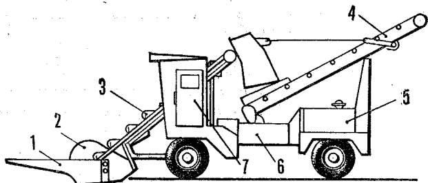
Рис. 1. Схема переоборудованного погрузчика: 1 — самоподающий лоток, 2 — винтовой шнек, 3 — ковшовой элеватор, 4 — ленточный транспортер, 5 — двигатель, 6 — топливный бак, 7 — кабина.
