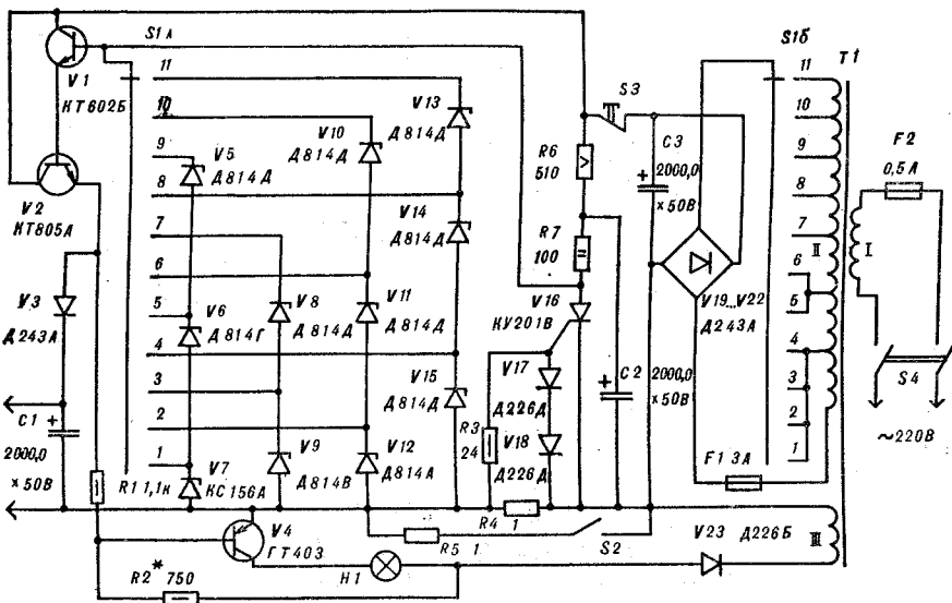
Рис. 1. Принципиальная схема источника питания.
