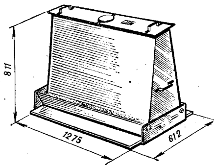
Рис. 7. Самокормушка для птицы и ее схема.
