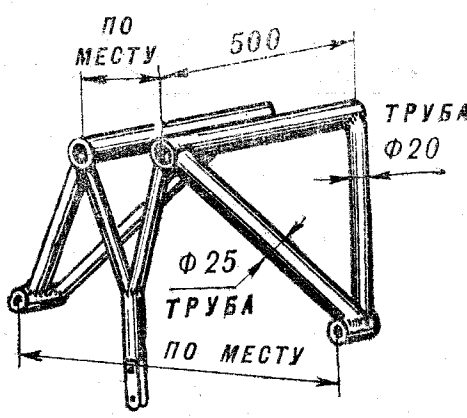
Рис. 4. Конструкция и основные размеры подмоторной рамы.
