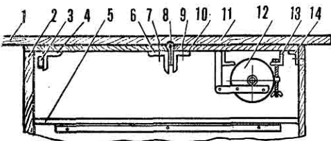
Рис. 4. Разрез тумбочки закрытого стола (вид справа):
