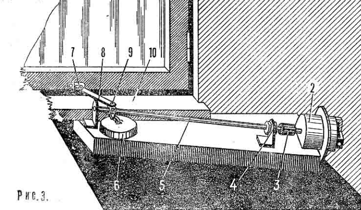
Рис. 2. Датчик-ванна: 1 — карниз подоконника, 2 — электролитическая ванна, 3 — прокладки (диэлектрик), 4 — винты крепления, 5 — электрод I, 6 — электрод II. Рис. 3. Привод: 1 — окно, 2 — электродвигатель, 3 — муфта (резиновая трубка), 4 — радиальноупорный подшипник, 5 — червячный вал, 6 — конечный выключатель, 7 — шарнир, 8 — тяга, 9 — ползунок.
