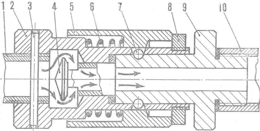
Рис. 3. Патрон для пневмомагистрала:
