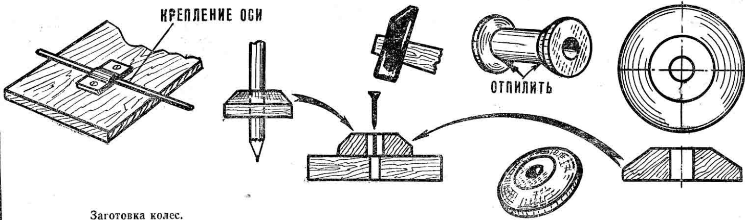
Заготовка колес.
