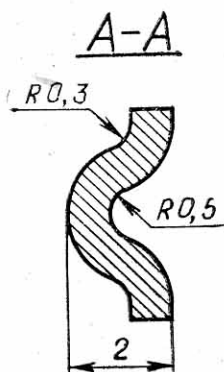
Рис. 4. Токопроводящие переходные стойки.
