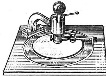
Рис. 4. Устройство для быстрого «раскроя» шлифшкурки.
