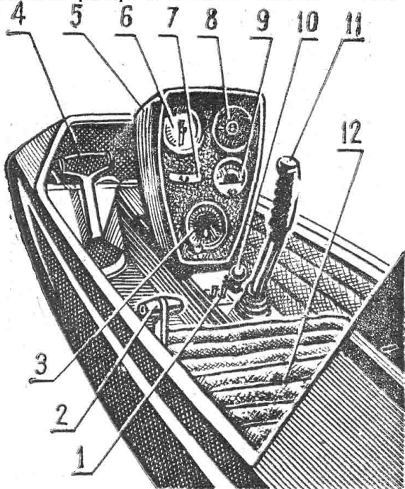
Рис. 3. Оборудование кабины: 1 — тумблеры электросистемы, 2 — газовый сектор, 3 — высотомер, 4 — педали управления рулем поворота, 5 — кожух блока приборов, 6 — указатель скорости, 7 — указатель поворота и скольжения, 8 — вариометр, 9 — тахометр, 10 — замок фонаря, 11 — ручка управления, 12 — сиденье пилота.
