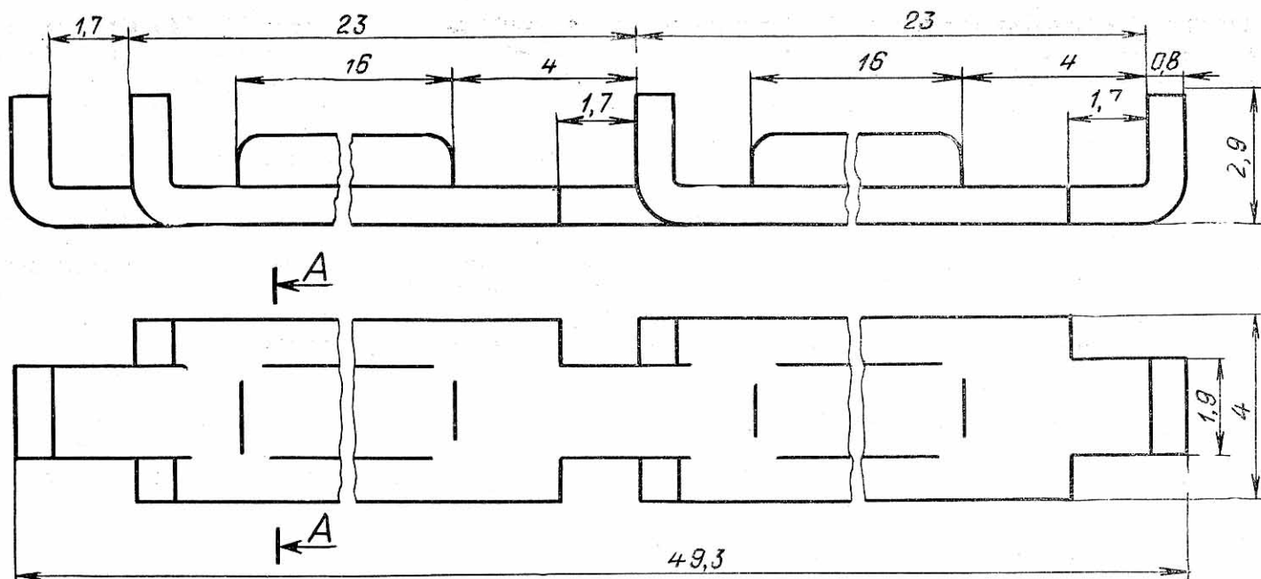
Рис. 4. Токопроводящие переходные стойки.
