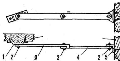
Рис. 7. Складной упор крышки стола в сборе:
