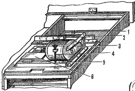
Рис. 3. Вид тумбочки с откинутой задней половиной крышки:
