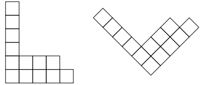
Рис. 4. Диаграммы Юнга
