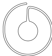
Р и с. 5. Сфера с экватором
