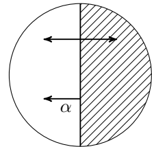
Рис. 2. Проективизация конуса
