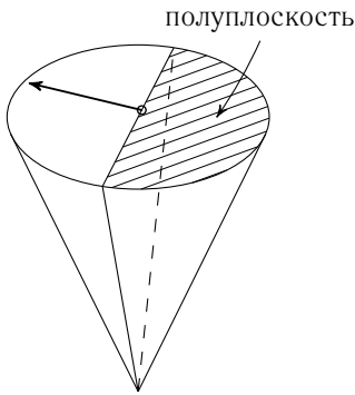
Рис. 1. Световой конус
