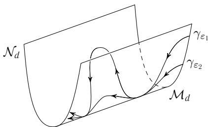
Рис. 5. Конфигурационное пространство
