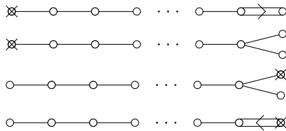
Р и с. 2. Диаграммы Дынкина для Q_n (первые две), OGr и LGGr
