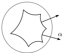
Рис. 3. Камера Вейля
