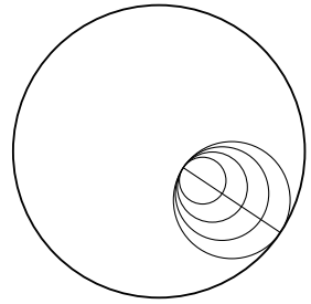
Р и с. 1. Орисфера
