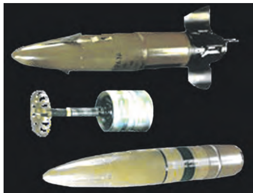
Управляемая ракета 9М119М «Инвар» для 125-мм танковых пушек
