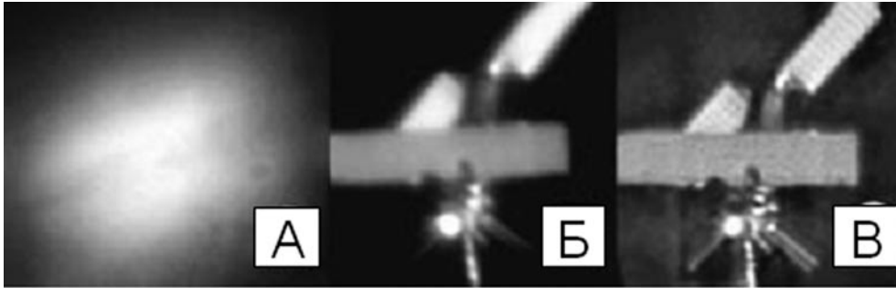
Изображение низкоорбитального КА, полученного в ходе испытаний АОС: А – без применения АОС, Б – с применением АОС и коррекцией в режиме реального времени, В – после компьютерной обработки
