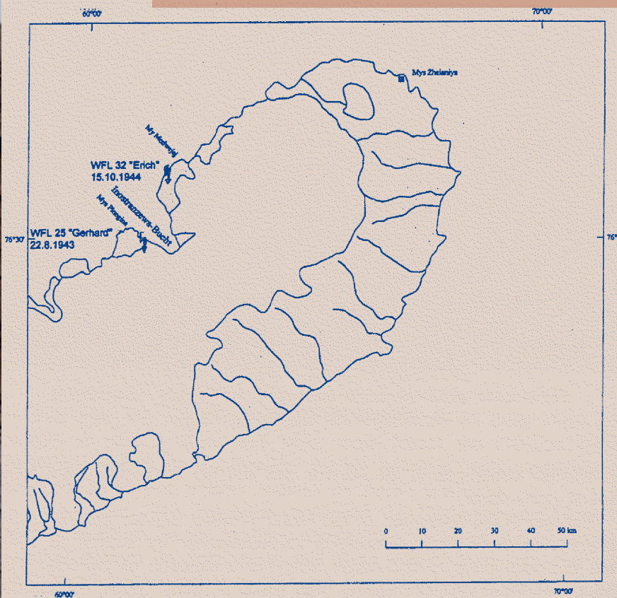
▲ Расположение автоматических метеостанций «W.F.L.» на Новой Земле с 22.08.1943 по 15.10.1944 гг. («Война в Арктике. 1939–1945 гг.». Архангельск, 2000)
