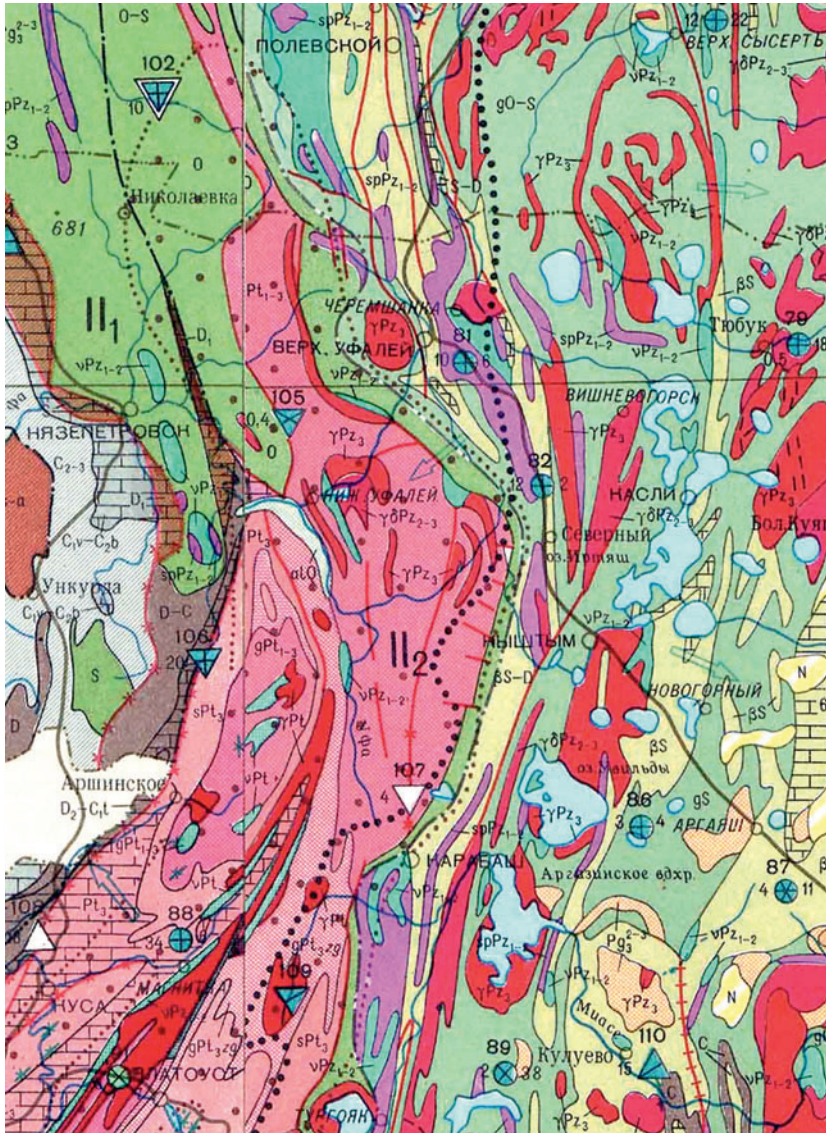
◀ Фрагмент геологической карты Урала
