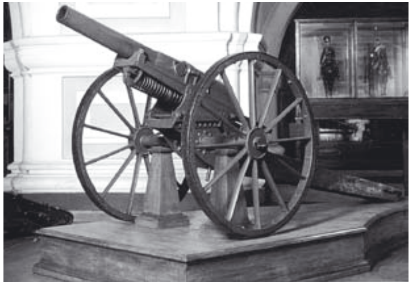
2,5-дюймовая скорострельная пушка В.С. Барановского обр. 1877 г. на упругом лафете.
