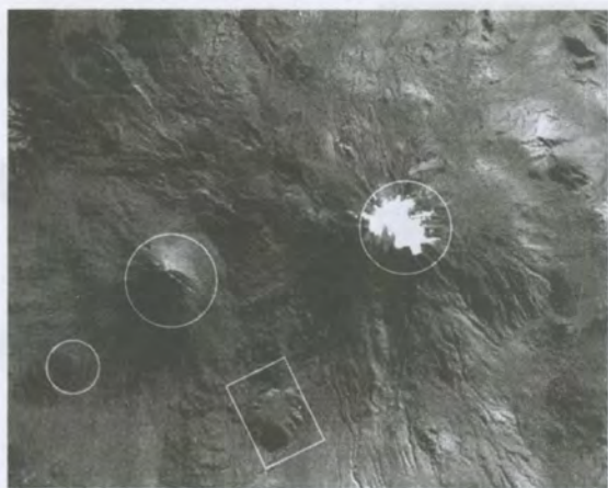
Араратский горный массив (вид сверху)
