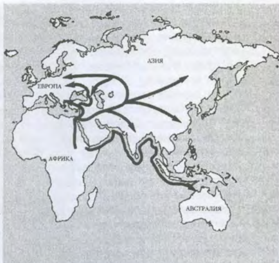
Схема предполагаемого расселения Homo Sapiens из Африки
