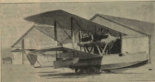
Летающая лодка С. А. М. S с двумя моторами Испано-Сюма по 275 лощ. сил каждой. Колеса под лодкой служат лишь для выката лодки из воды на сушу.
