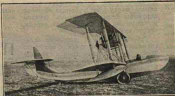
Гидро-самолет „Амфибия“ Е. В. А. 17 с мотором Испано-Сюма, 180 лощ. сил.
