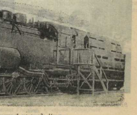
Локомотив с турбиной, построенный на заводе Круппа.
