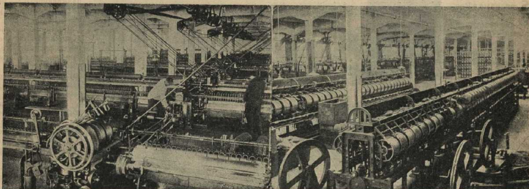
П РАДИЛЬНОЕ ОТДЕЛЕНИЕ: Соельфактора.
