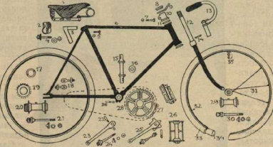
1. Седло. 2. Замок для седла. 3. Седельный крок. 4. Болт для крепления седла. 5. Болт для крепления седельного крока к раме. 6. Педаль. 7. Болт рулевой колонки. 8. Конторайка. 9. Формы крок. 10. Колпачок рулевой. 11. Вилка воловчатая чашка. 12. Передняя вилка. 13. Руль. 14. Нижняя воловчатая чашка. 15. Ось каретки. 16. Чашка каретки. 17. Конторайка задний втулки. 18. Нижняя для цепи с вилками. 19. Задняя малая шестерня. 20. Задняя втулка. 21. Задний вал. 22. Педальная ось с вилкой и конусом. 23. Килька для втулок с вилками. 24. Педальная ось с вилкой, шайбой и конусом (левая). 25. Правый шатунок. 26. Педаль. 27. Цепь. 28. Средняя большая шестерня. 29. Передняя втулка. 30. Передняя ось с вилкой, шайбой и конусом. 31. Спицы. 32. Обод. 33. Покрышка. 34. Камера. 35. Вентиль. 36. Болты для крепления чашек.
