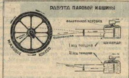
ЗОЛОТНИКОВАЯ КОРОБКА: на первом ходу паровоза пар попадает в правую часть цилиндра и толкает поршень влево. Когда он сойдет до конца, коробка автоматически подает пар в левую часть цилиндра, что заставляет поршень двинуться вправо.
