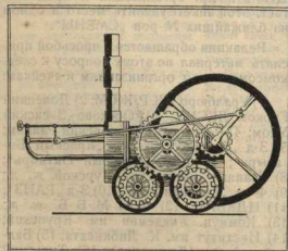
ПРАДЕДУШКА СОВРЕМЕННОГО ПАРОВОЗА локомотива Тревитика (1804). В нем интересна передача движения маховика на колеса посредством зубчатых колес.
