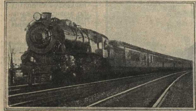
СЛЕВА: АМЕРИКАНСКИЙ ЭКСПРЕСС (скорый поезд) Чикаго-Нью-Йорк. СПРАВА: СХЕМА УСТРОЙСТВА ПАРОВОЗА: вода в котле, нагревая топкой А, превращается в пар, который собирается в верхней части локомотива, и за счет по трубе Д идет в золотниковую коробку Е. Коробка распределяет пар в цилиндры, заставляя его двигать поршень и соединенный с ним козлун Ж и шатуны З, вращающие колеса.
