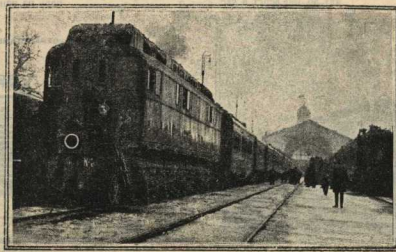
ТЕПЛОВОЗ ГАККЕЛЯ; в бокалах Октябрьской ж. д. в Москве перед встречей.
