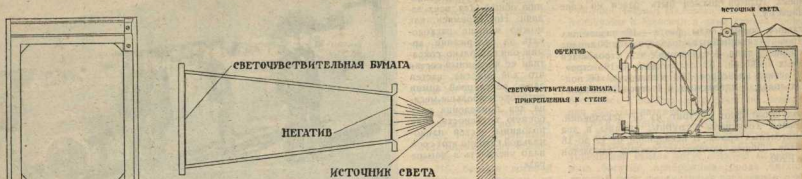
В СЕРЕДИНЕ: Схема устройства камеры для увеличения. СЛЕВА: матовое стекло, которое нужно вынуть и аппарат. СПРАВА: Общий вид домашней установки для увеличения снимков.
