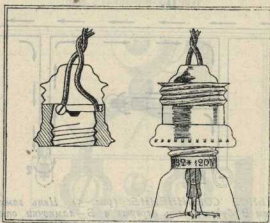
Разрез и внешний вид патрона электрической лампочки.
