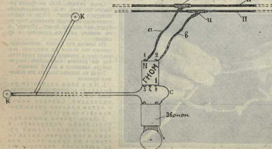
СХЕМА ПРОВОДКИ ЭЛЕКТРИЧЕСКОГО ЗВОНКА БЕЗ ЭЛЕМЕНТОВ: ПП — проводка осветительной сети; ИИ — место присоединения отвода «а» и «б»; цифры 1, 2, 3, 4 и 5 — проводки к зажимам трансформатора «Гном»; КК — кнопки.
