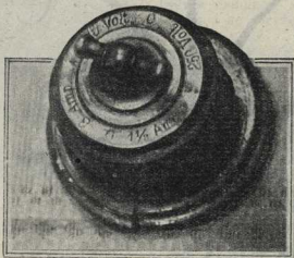
ВЫКЛЮЧАТЕЛЬ ДЛЯ ЭЛЕКТРИЧЕСКОГО ОСВЕЩЕНИЯ. На снимке не видно входящей в него проводки; она проложена по обоим и выходит в выключатель снизу.
