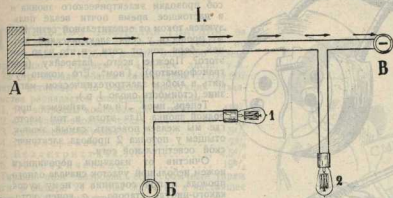
ПОСЛЕДОВАТЕЛЬНОЕ СОЕДИНЕНИЕ: (рис. 3). Повернутый выключатель В не зажегнет лампочек, потому что цепь не замкнута выключателем В. Стрелки показывают путь тока.
