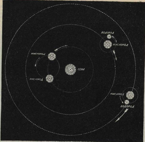
СХЕМА МОЛЕКУЛЫ СЕРНОЙ КИСЛОТЫ, состоящей из двух атомов водорода, одного атома серы и четырех атомов кислорода (H 2 SO 4 ). На схеме показаны пути движения атомов и электронов, из которых составлен каждый атом.
