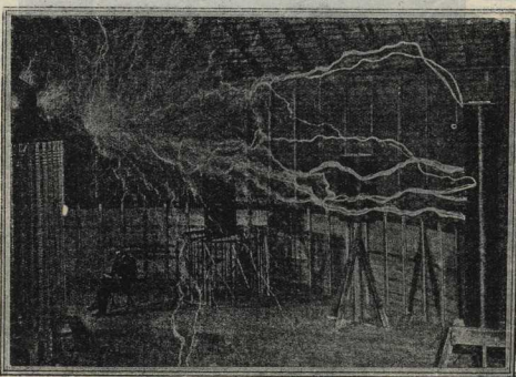
ВЕЛИЧАЙШАЯ ИСКУССТВЕННО ДОБЫТЫЕ ЭЛЕКТРИЧЕСКИЕ ИСКРЫ. Она получена американцем Телес в его лаборатории, близ Колорадо, Америка.
