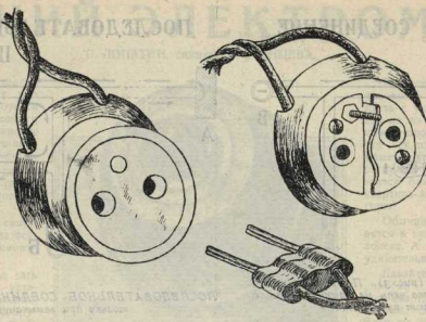
ШТЕПСЕЛЬ И ВИЛКА ДЛЯ ПЕРЕНОСНЫХ ЛАМП: Слева — разрезное гнездо штепселя, на котором видна предохранительная проволочка.
