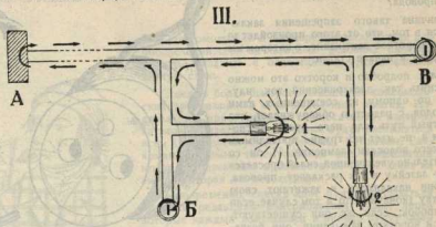
ПОСЛЕДОВАТЕЛЬНОЕ СОЕДИНЕНИЕ: (рис. 4). Они загорятся только при замыкании обеих выключателей.
