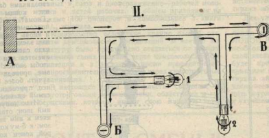
ПОСЛЕДОВАТЕЛЬНОЕ СОЕДИНЕНИЕ: (рис. 5). Цепь замкнутая одним выключателем В будет иметь прерыва в В — лампочки опять не могут гореть.
