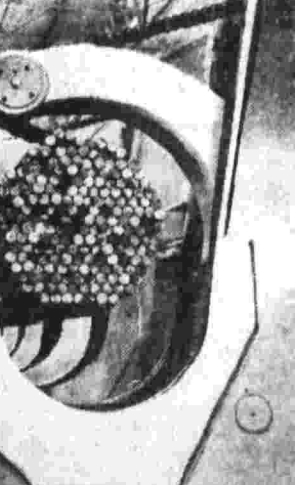
В сотрудничестве с металлургами Крюкова Рог и Новокузнецка на народном предприятии тяжелого машиностроения — комбинате Искра в г. Магдебурге создано это устройство для панкратирования прутков стали. Оно изготовлено с помощью прутки стали длиной до 6 метров в пакете весом по 8,5 тонны.
