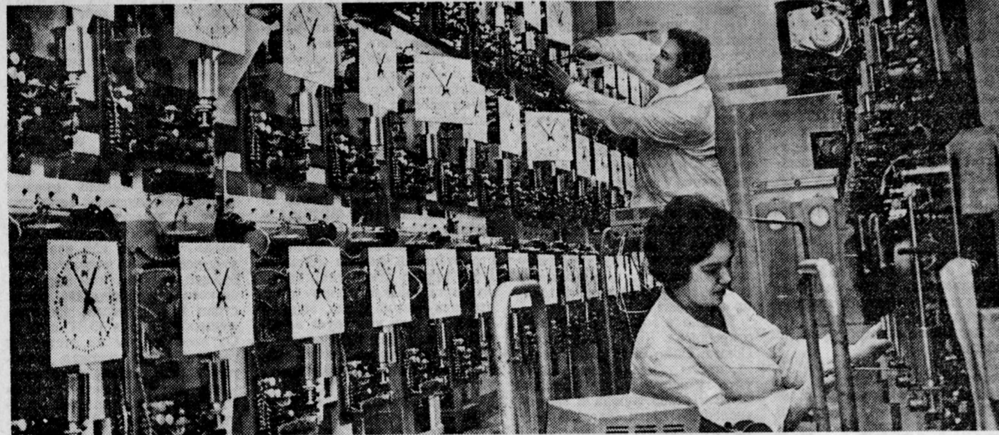
ЛЕНИНГРАДСКИЙ завод электрочасов выпускает около 40 видов изделий. Реле времени, печатные хронографы, электрочасовые меры и многие другие приборы изготавливаются в заводских цехах. Собирают их мастера и ученики в цехах. Фото В. Самойлова.
