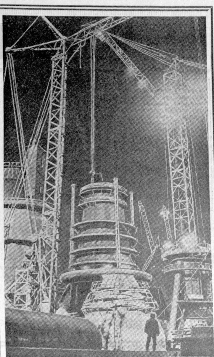
НА СТРОИТЕЛЬСТВЕ четвертой доменной печи Орско-Халиловского металлургического комбината в Оренбургской области горячая пора. Участвуя во Всесоюзном социалистическом соревновании за досрочное выполнение плана 1973 года, пятилетний коллектив строителей и монтажников решил сдать дому в эксплуатацию на двадцать дней раньше срока, 10 декабря этого года. Новая печь во всем покажет себя превзойдет действующую на комбинате. На снимке вверху — победители социалистического соревнования члены бригады монтажников В. Ветчинкина устанавливают знамя на самой высокой точке печи № 4; вверху — днем и ночью идет монтаж четвертой доменной. Фото Н. Кузнецова (ТАСС).
