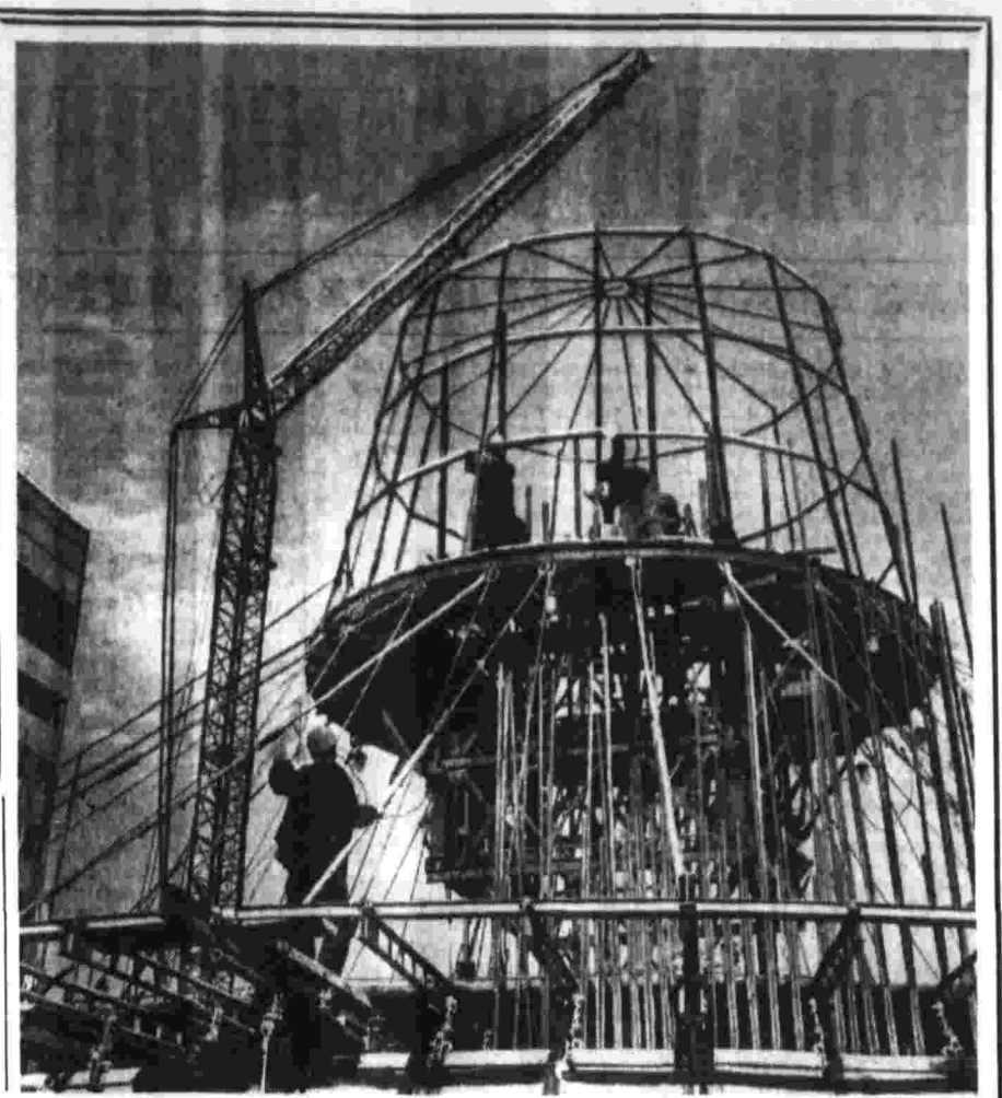
Недавно пущен третий энергоблок мощностью 300 тысяч киловатт на Иринлинской ГРЭС — всеосознанной ударной московской стройке. На очереди — установка четвертого энергоблока такой же мощности. Началась строительство 220-метровой дымовой трубы для этого агрегата. На с ним идет монтаж оплывающей дымовой трубы. Фото Н. Кузнецова (ТАСС).
