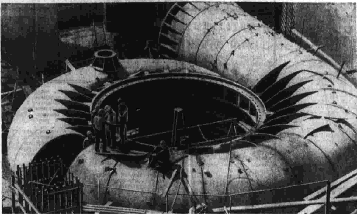
Таджикская ССР. Нурунская ГЭС — сердце Южно-Таджикского территориально-производственного комплекса, создаваемого по Директивой XXIV съезда КПСС. Здесь готово основание для всех девяти гидротурбин. Мощность каждой из них — 300 тысяч киловатт. На гидроагрегате № 9 сейчас идет подготовка и испытание спиральной камеры гидравлическим давлением. Фото Ю. Угрюмова. (ТАСС).
