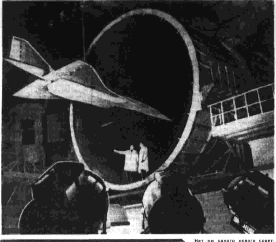
Нет ни одного нового советского самолета, который не прошел бы аэродинамических исследований в Центральном аэродинамическом институте. И с ним же: подготовка и испытание аэродинамической трубе модели сверхзвукового пассажирского лайнера ТУ-144. Фото И. Гричера.
