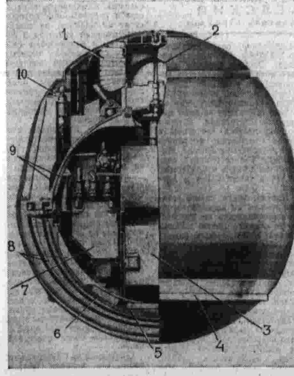
СПУСКАЕМЫЙ АППАРАТ «ВЕНЕРА-7»: 1 — парашют; 2 — передняя антенна; 3 — радиопередатчик; 4 — опорное кольцо; 5 — демфер; 6 — силовой корпус; 7 — блок коммутации; 8 — теплозащитная; 9 — теплообменник; 10 — крышка парашютного отсека.
