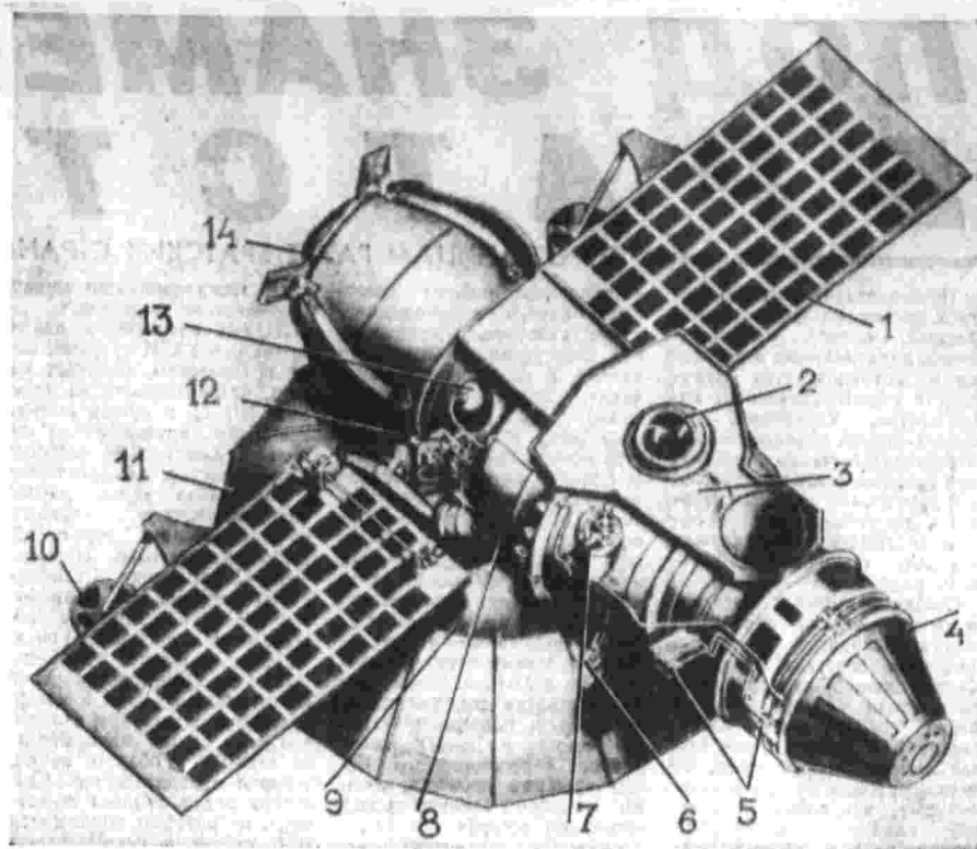
МЕЖПЛАНЕТНАЯ АВТОМАТИЧЕСКАЯ СТАНЦИЯ «ВЕНЕРА-7»: 1 — панели солнечных батарей; 2 — датчик астроориентации; 3 — защитная пленка; 4 — корректирующая двигательная установка; 5 — коллекторы пневмосистемы с управляющими соплами; 6 — свечки космической части; 7 — датчик постоянной солнечной ориентации; 8 — орбитальный отсек; 9 — радиатор-охладитель; 10 — малонаправленная антенна; 11 — остронаправленная антенна; 12 — блок автоматической пневмосистемы; 13 — баллон сжатого азота; 14 — спускаемый аппарат (СА).
