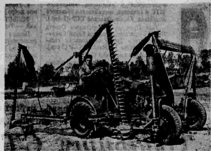
На выставке механизации животноводческих ферм. На снимке: самоходная сенокосилка «КС-10» конструкции Всесоюзного научно-исследовательского института механизации и электрификации сельского хозяйства, выпущенная Люберецким заводом.
