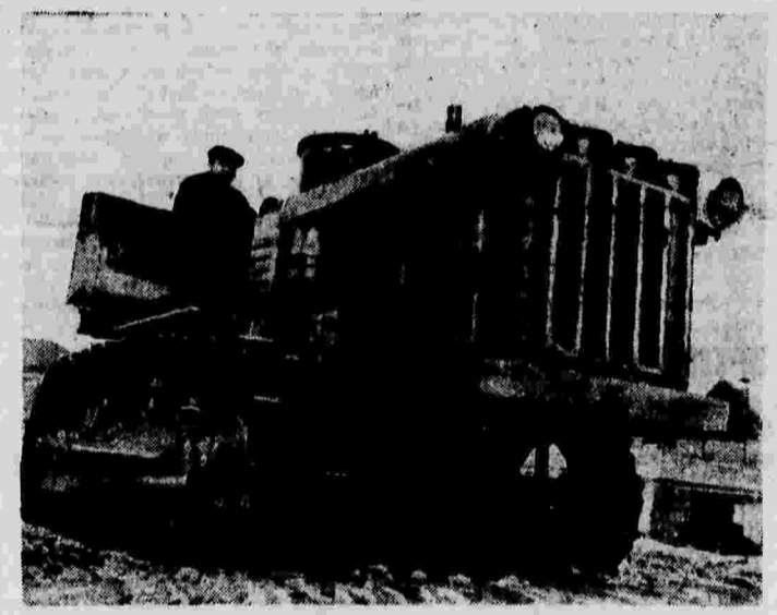
Обкатка одного из первых газогенераторных тракторов на Челябинском тракторном заводе им. Сталина. Фото В. Ташчанина (Совзнаго).
