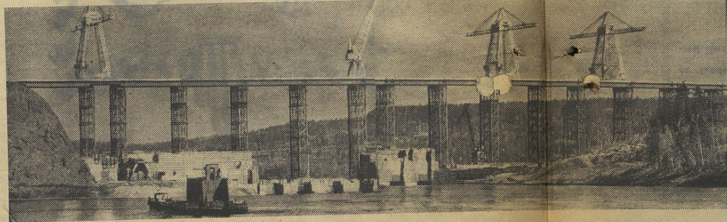
Новая гигантская стройка в Сибири — Усть-Илимская ГЭС. Сегодня здесь работают комсомольцы, чьи отцы строили Магнитку, Комсомольск на Амуре, Днепродзержинск. Фото ТАСС.
