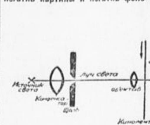
Рис. 1. Схема воспроизведения звука.
