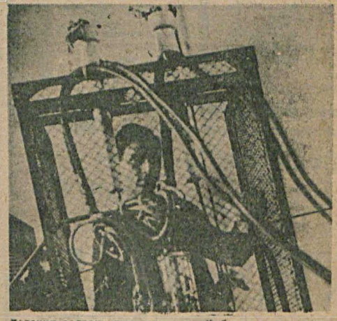
Догенили заграничную технику. Лаборатория завода «Светлана» в Ленинграде закончила испытание генераторных радио-ламп, мощностью в 200 квт. Новые лампы являются одними из самых мощных в мире. На снимке: установка на испытание первой советской лампы в 200 квт.
