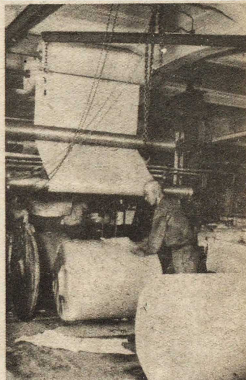
На Балачинской бумажной фабрике. Бумага в роллах
