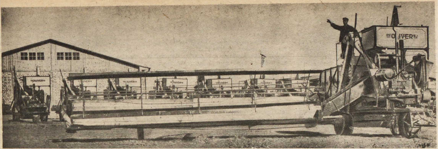
В совхозе „Гигант“ Сев.-Кав. края. Комбайн „Оливер“ перед выездом на участок
