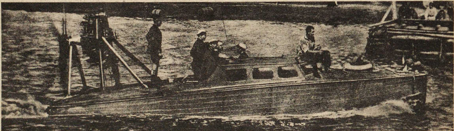
Поход глассеров Москва—Астрахань является генеральной проверкой советских глассерных конструкций. На снимке — глассер им. Сталина в пути. Фот. И. Шагина
