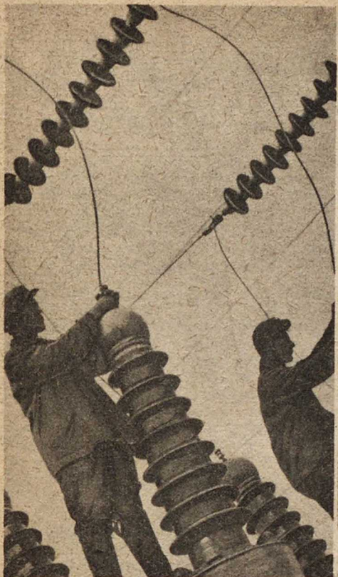
Монтаж открытой подстанции Нижегородского автозавода, законченной на три дня раньше срока Фот. И. Канелюша
