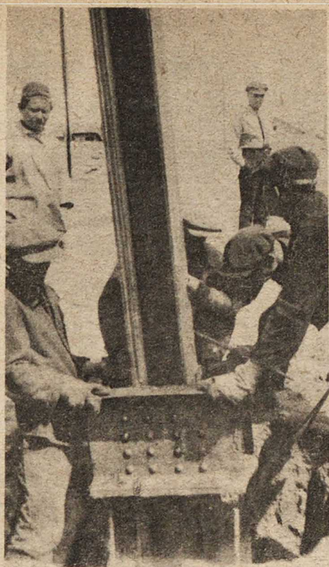
На строительстве Челябинского тракторного завода. Ударная бригада монтажников на креплении конструкций к фундаментам
