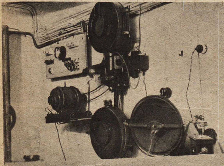
Звуковоспроизводящий аппарат системы „тагелефон“
