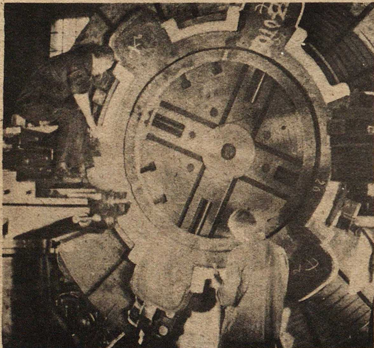
Ленинградский завод «Электросила» выполняет заказ Магнитостроя на поставку генераторов и электромоторов. На снимке: ударная бригада им. Магнитостроя за обточкой станины генератора
