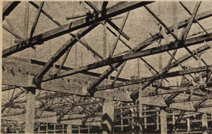
Строящийся деревообделочный цех сибирского завода комбайнов (Ново-Сибирск)
