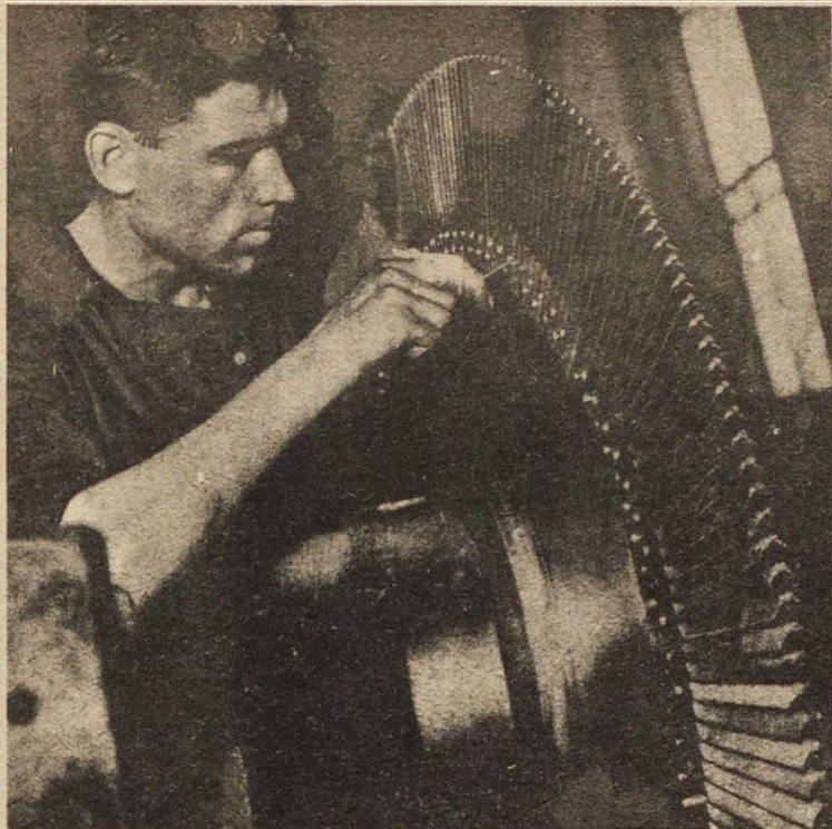
Донецкий завод им. Сталина выпустил впервые в СССР сварной конденсатор для турбины в 24 тысячи киловатт. Конденсатор такой мощности был лишь однажды изготовлен два года тому назад на одном из американских электровзводов и при испытании дал течь. Испытание, произведенное с конденсатором, выпущенным заводом им. Сталина, показало его высокие качества и полную годность. На с л и м а х и с т е в а — ударник на обрзотной ротора; с п р а в а — балансировка ротора колеса Пельтона (гидравлическая турбина) Фот. А. Шайкета
