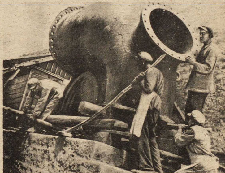
На Дзержинском (Армения, Эривань) заканчиваются строительные работы. На снимке: выгрузка частей турбины, изготовленной ленинградским заводом крупного машиностроения
