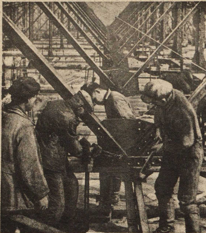
Заклепка конструкции в мартеновском цехе
