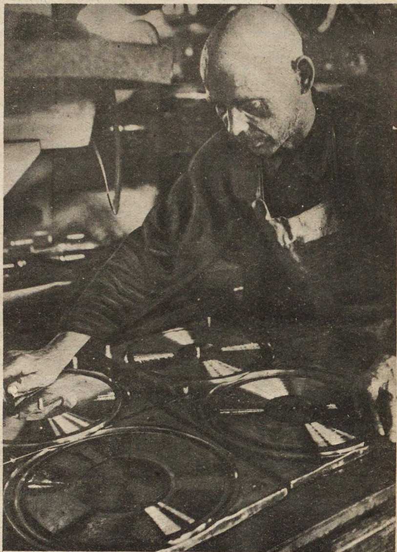
Прессовка граммофонных пластинок. Прессовщик протирает матрицу Фот. М. Вуколова
