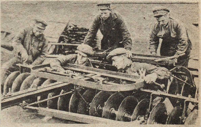
На заводе «Сельмаш» в Ростове-на-Дону. Комсомольская ударная бригада по сборке дисковых боров, дающая ежемесячно перевыполнение программы Фот. Ю. Дружелюбова
