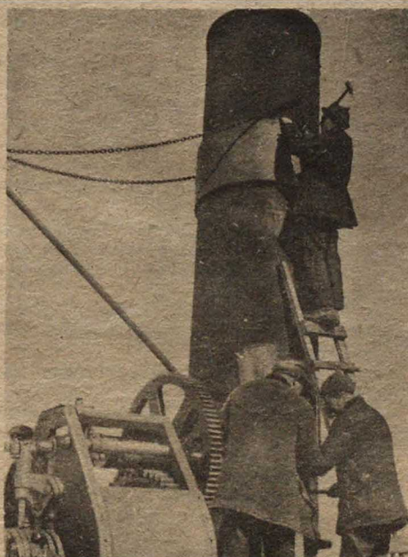
Установка и монтаж трубы на пароходе «Комсомолец» рабочими мастерских Днепровского госпредприятия
