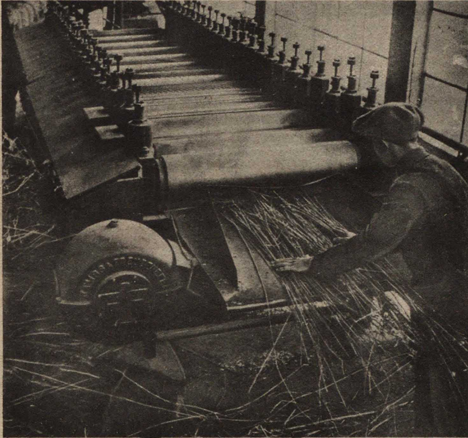
Опытная фабрика по обработке лубяных волокон. Работа декортикатора
