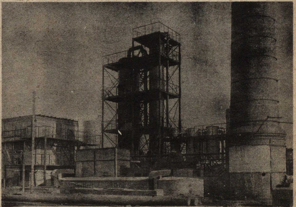
Банинские нефтяные заводы. Первый советский крекинг системы Жукова-Каполюшника
