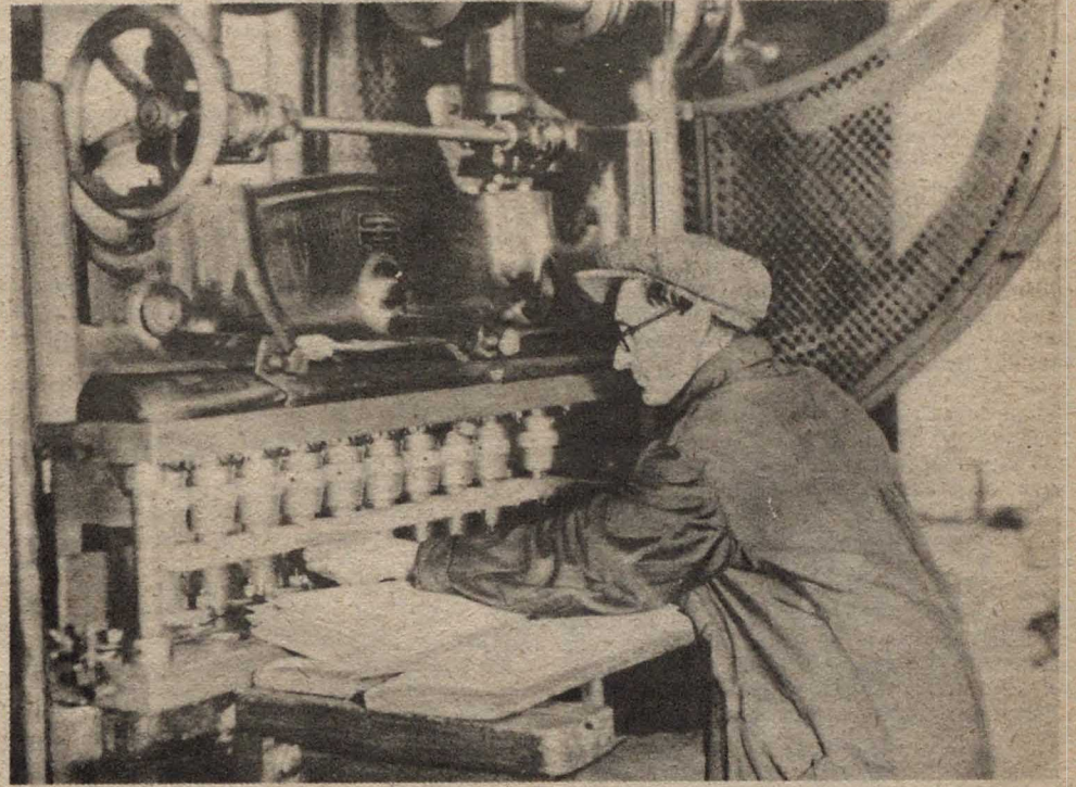
Опускание готового сердечника трансформатора в кожух
