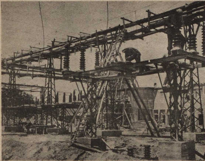
Стройка новой электростанции в с. Каспи. Монтаж воздушной линии
