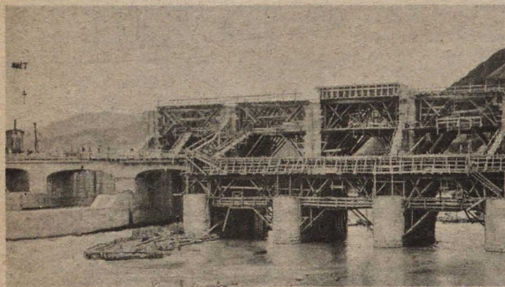
Десять лет Советской Грузии. Стройка годового сооружения РивГЭС
