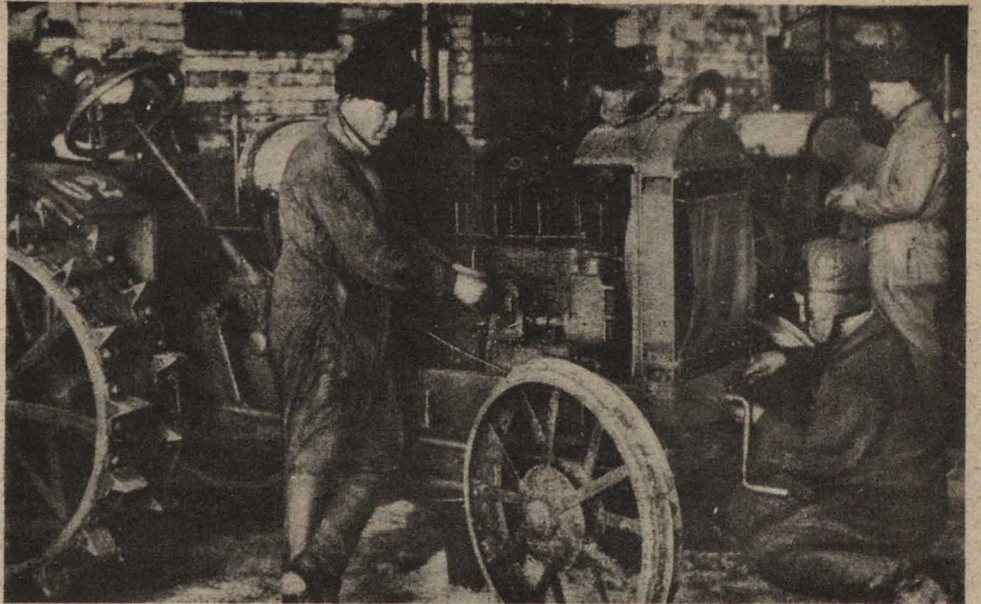
Ремонт тракторов и сель.-хоз. инвентаря в ремонтных мастерских колхоза „Гигант“ Сальского округа закончен. В ударном порядке ремонтируются тракторы для малоомощных колхозов Донецкого и Сальского округов
