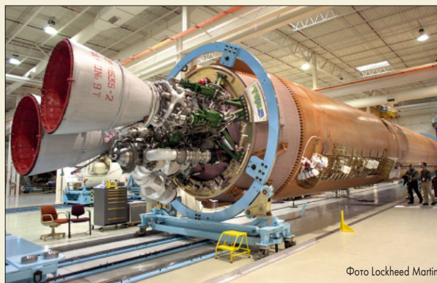
Центральный блок PH Atlas 5 в сборочном цеху компании Lockheed Martin
