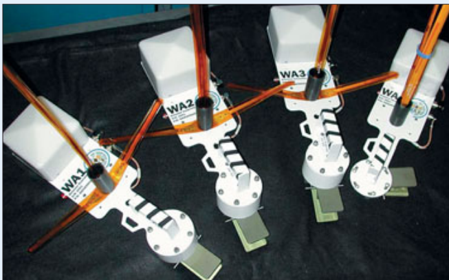
Антенны WA, предназначенные для установки на Агрегатном отсеке СМ
