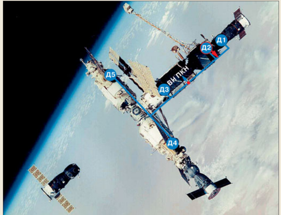
Схема расположения аппаратуры комплекса «Гермес» на борту ОК «Мир»: ВН – вычислитель негерметичности; ПКН – пульт контроля негерметичности; Д1...Д5 – аппаратура контроля негерметичности «Дюза-2М»
