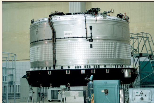
Сбрасываемый торовый бак разгонного блока «Бриз-М»
