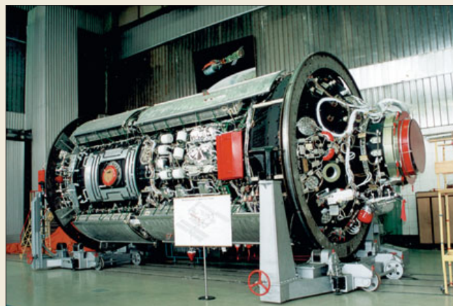
Модуль ФГБ-2
