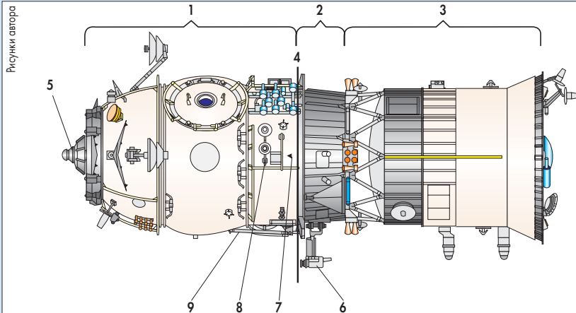
Грузовой корабль-модуль «Прогресс М-СО1»:
