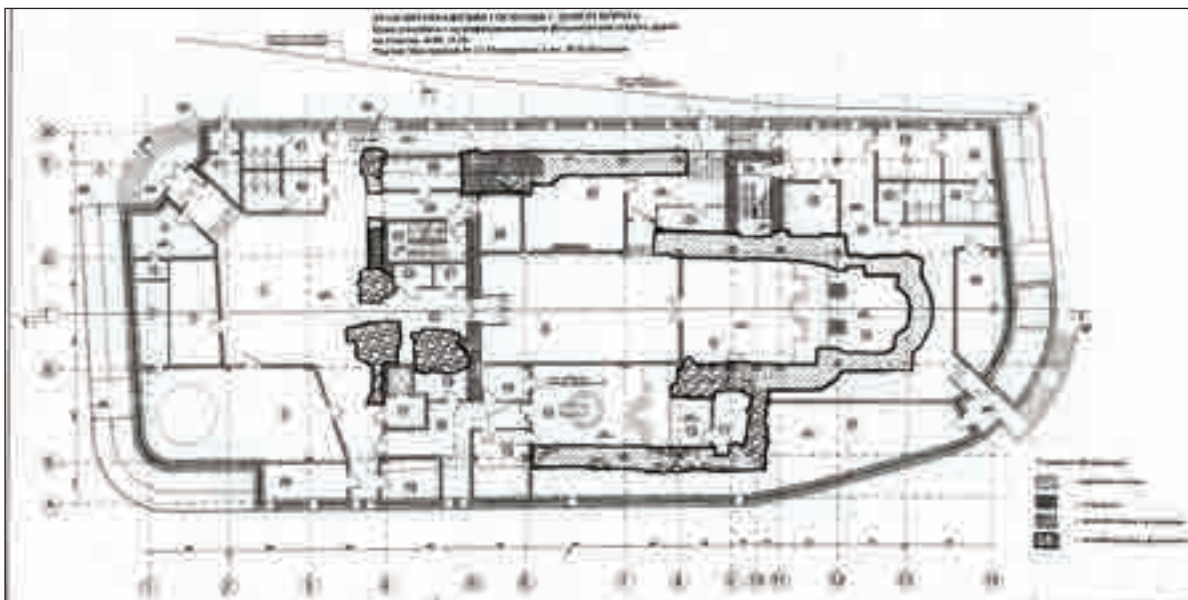
Чертеж стилобатной части храма с предлагаемыми для музеефикации историческими фундаментами. Проект
