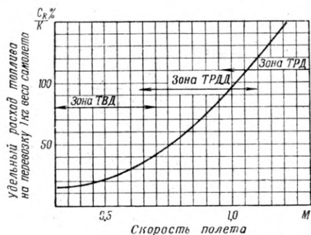
Рис. 4. Удельный расход топлива на перевозку 1 кг веса самолета в зависимости от скорости полета.
