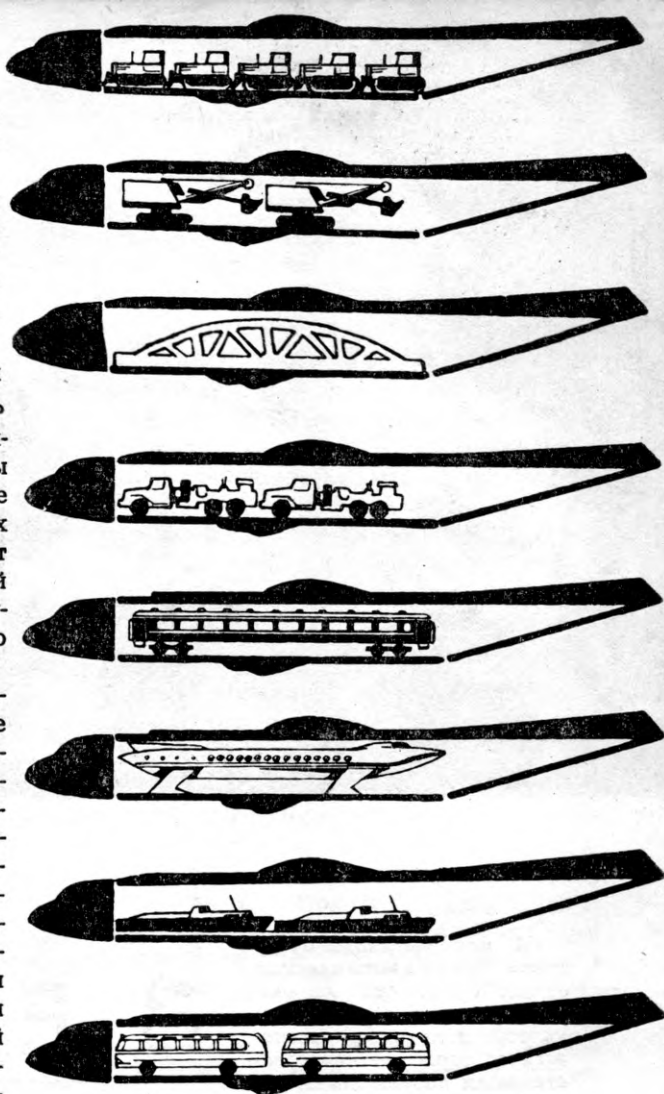
Рис. 8. Варианты загрузки самолета АН-22: 1 — Бульдозеры Д-535, 5 шт. по 6560 кг; 2 — Экскаваторы Э-656, 2 шт. по 22100 кг; 3 — Железобетонные фермы, 5 шт. по 12000 кг; 4 — Цементовый агрегат ЦА-300 для буровых работ, 2 шт. по 15500 кг; 5 — Пассажирский железнодорожный вагон, 49500 кг; 6 — Теплоход «Чайка», 14200 кг; 7 — Патрульное судно ПС-5, 2 шт. по 11400 кг; 8 — Междугородный автобус ЛАЗ-699А, 2 шт. по 7840 кг.
