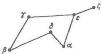
рис 2. Конфигурация звезд Большой медведицы 100 000 лет назад
